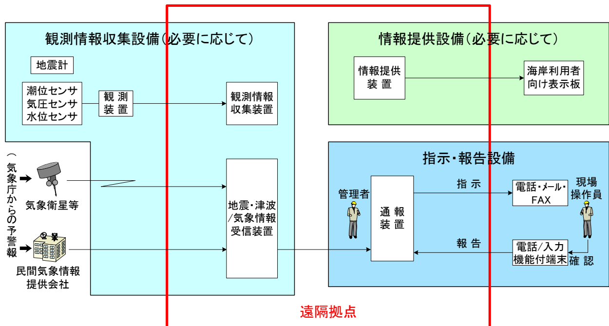
図 5.1-6 水門・陸閘等管理システムの設備構成例（システムレベル3）
