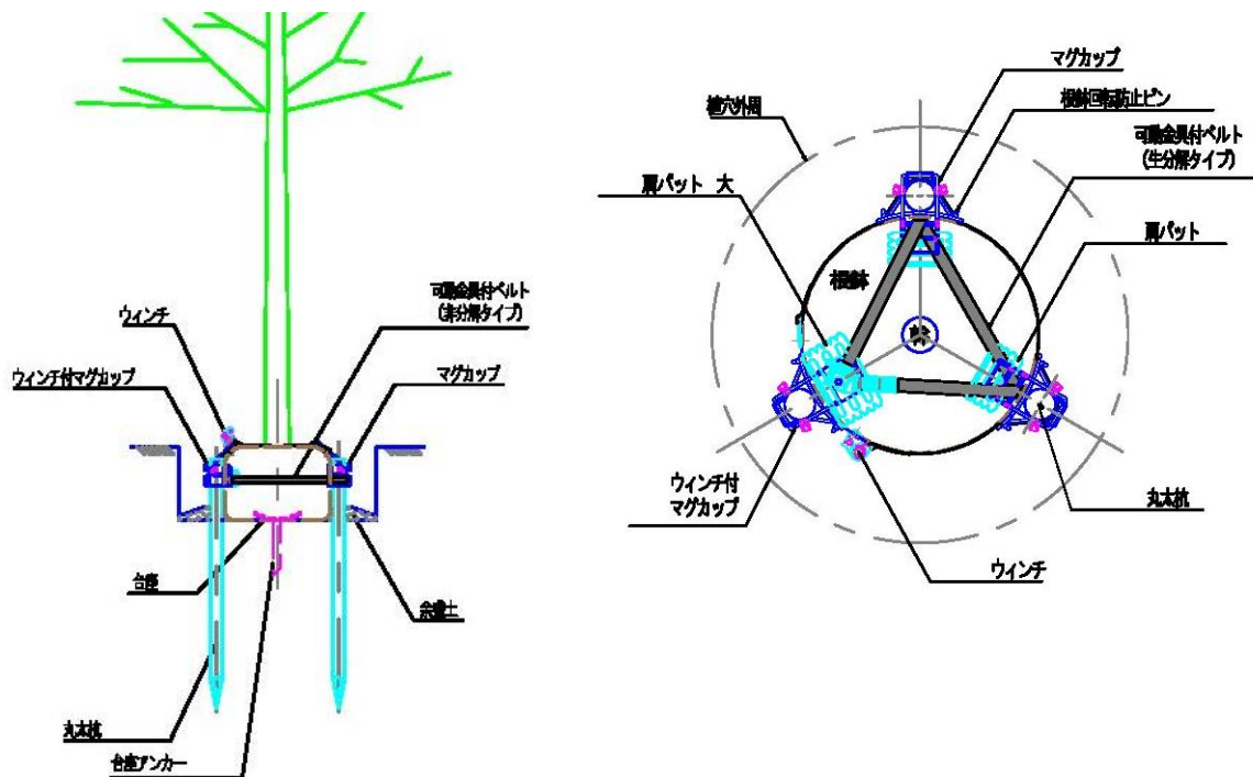
図-14 樹木へのアンカー設置（岐阜大学 原田守啓氏提供）
