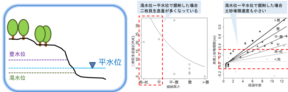
図 7 揖斐川における掘削高さと二枚貝、土砂堆積との関係 7)
