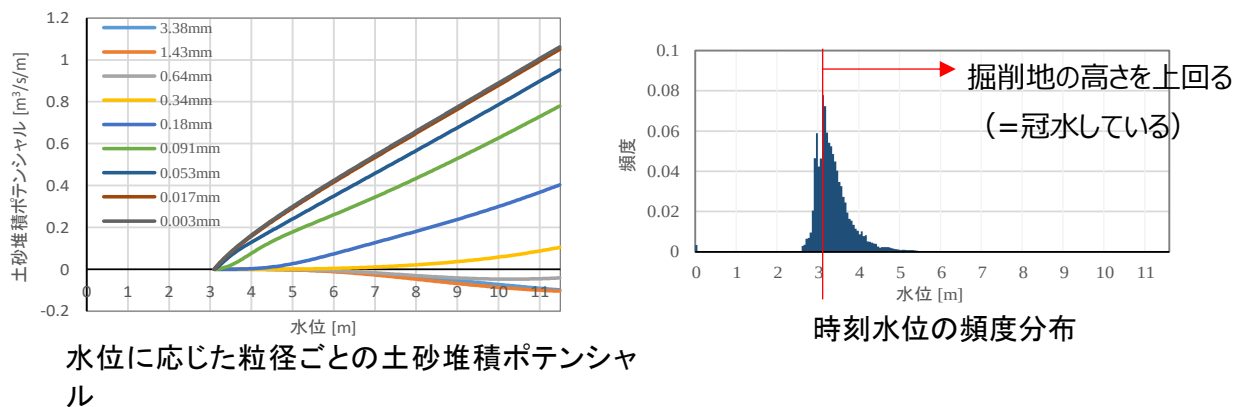
図 5 水位に応じた土砂堆積ポテンシャルと水位の時間頻度分布の例 5) より再作図
