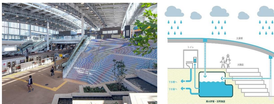
図 7-1 雨水利用施設の例（南町田グランベリーパーク駅）
