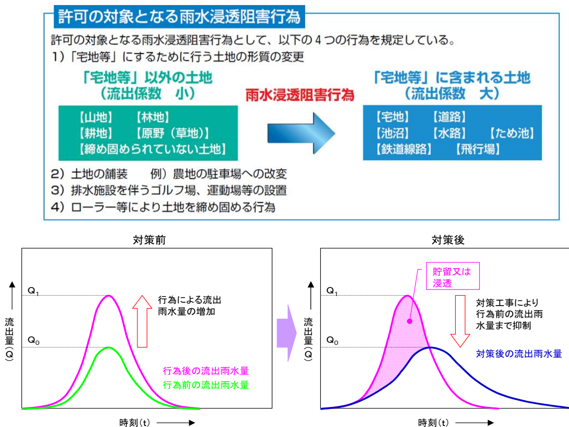
図 1-3 雨水浸透阻害行為と許可に必要な雨水貯留浸透施設のイメージ
