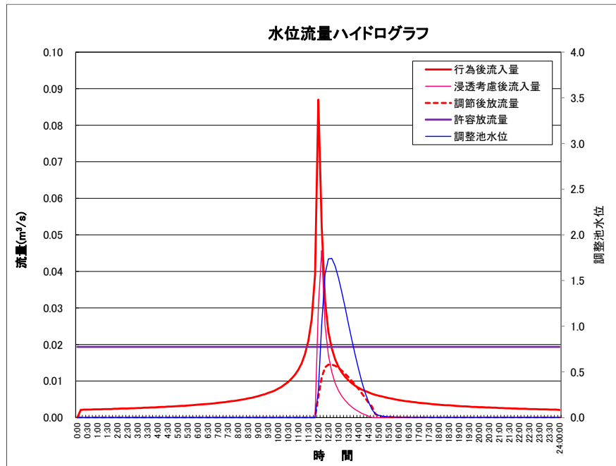
図 1-5 水位流量ハイドログラフ（調整計算シート）
