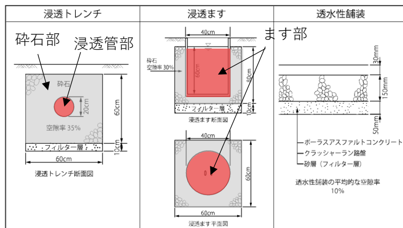
図 5-6 浸透施設の空隙貯留（一般概念図）
