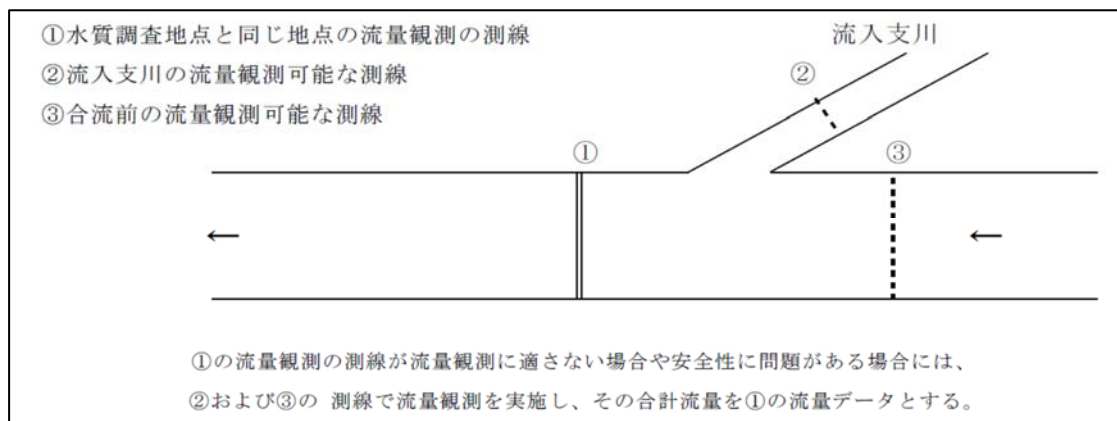
参考図1 合流部における流量観測の調査測線の設定方法の一例
