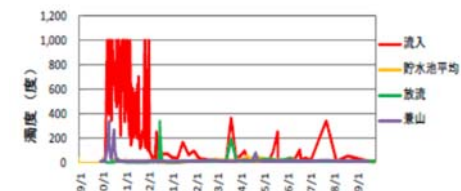
図-2 噴火後の濁度の変化
