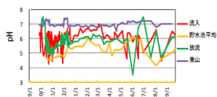
図-3 噴火後のpHの変化
