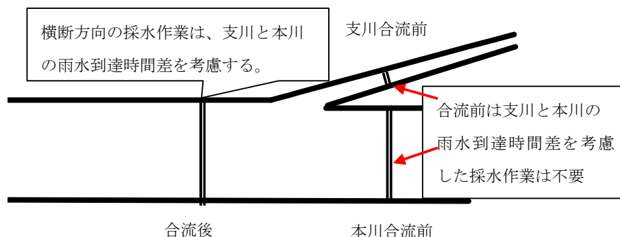
図 2.1 合流点付近の調査地点選定時の工夫
