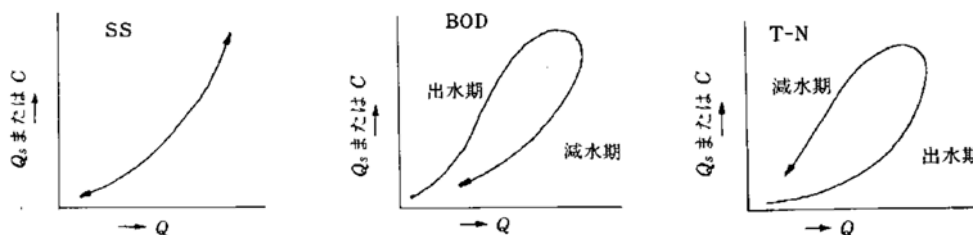
図 2.2 出水時の流量増加に伴う水質濃度Cまたは負荷量 Q_s の関係
