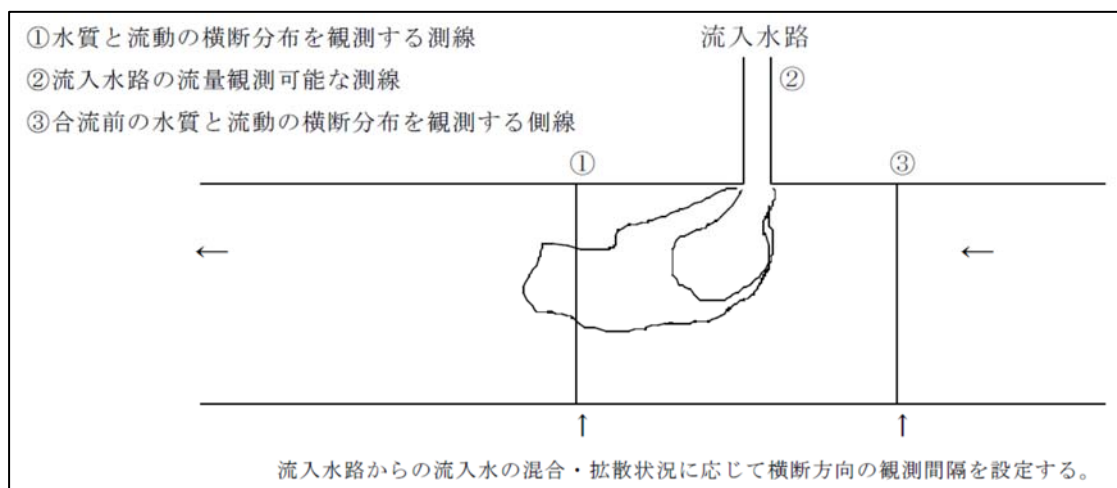
参考図2 横断方向の流動の調査地点（水質解析用）の一例
