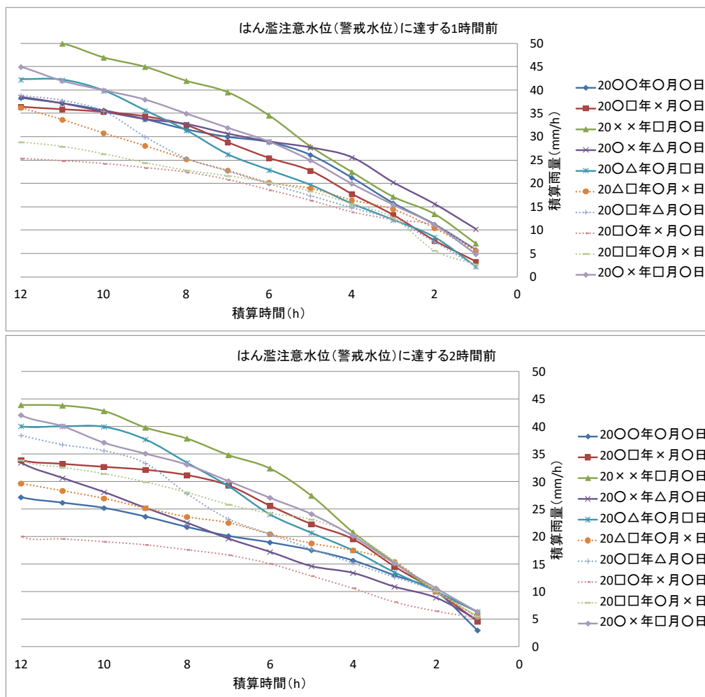
図一■ 氾濫注意水位（警戒水位）に達する1時間前、2時間前までの積算雨量
