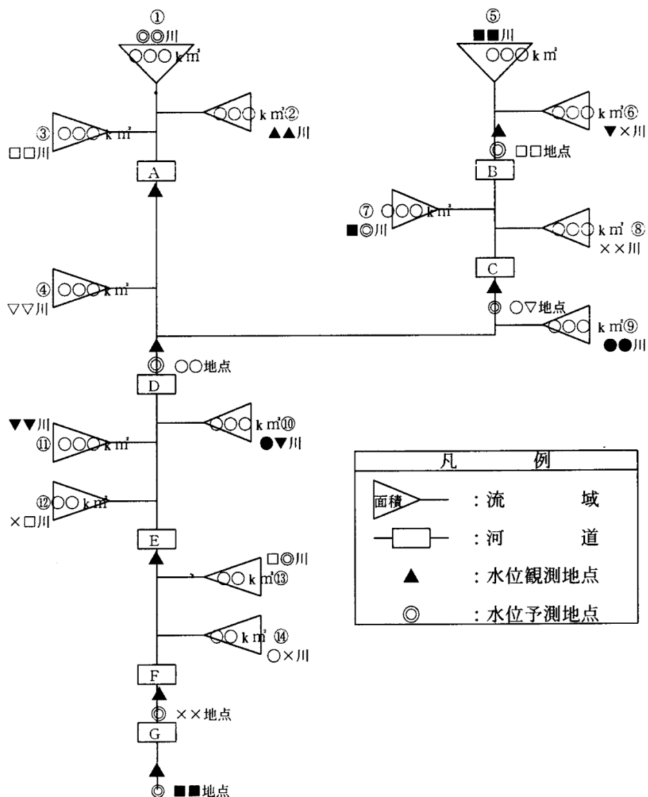
図一 ■ ○○川流出計算系統図
