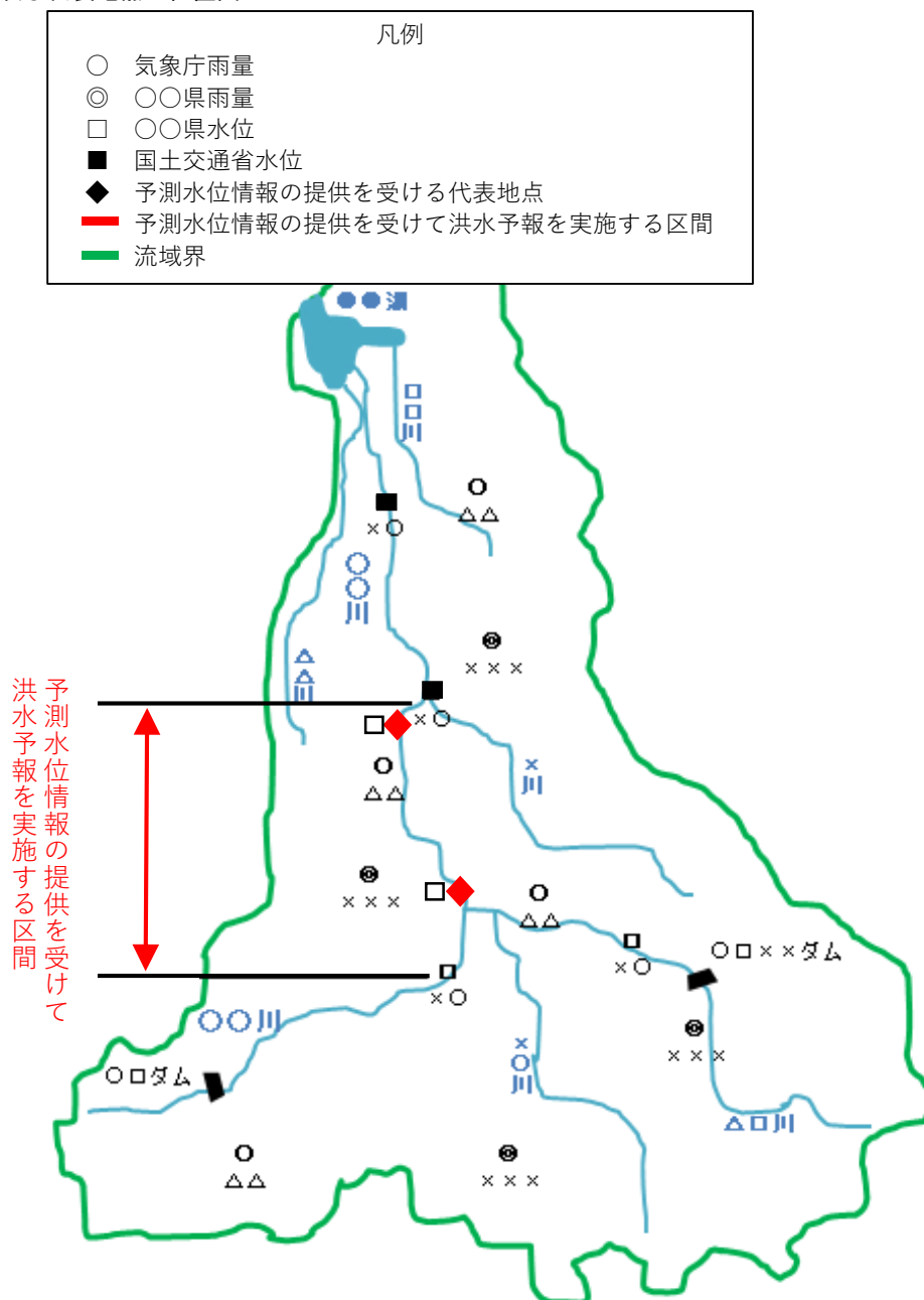
付図1 洪水予報区間及び雨量・水位観測所、並びに〇〇地方整備局から予測水位情報の提供を受ける河川・区間及び代表地点の位置図
