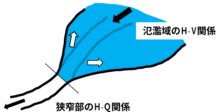
図 4-4 池モデルのイメージ図
