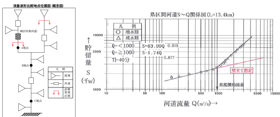
図 4-7-1 氾濫を考慮する場合と考慮しない場合の感度分析のイメージ図
