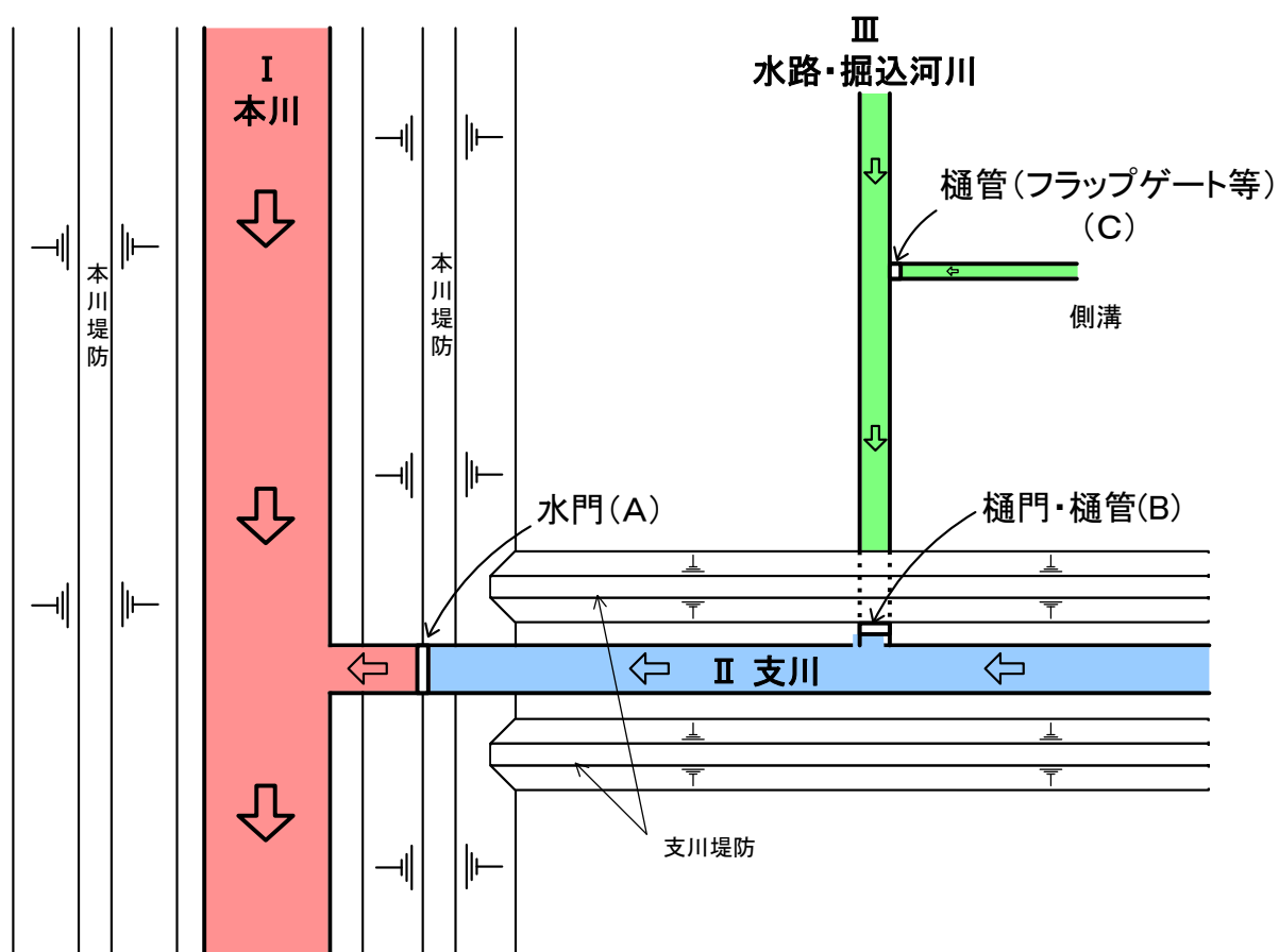
想定平面図
