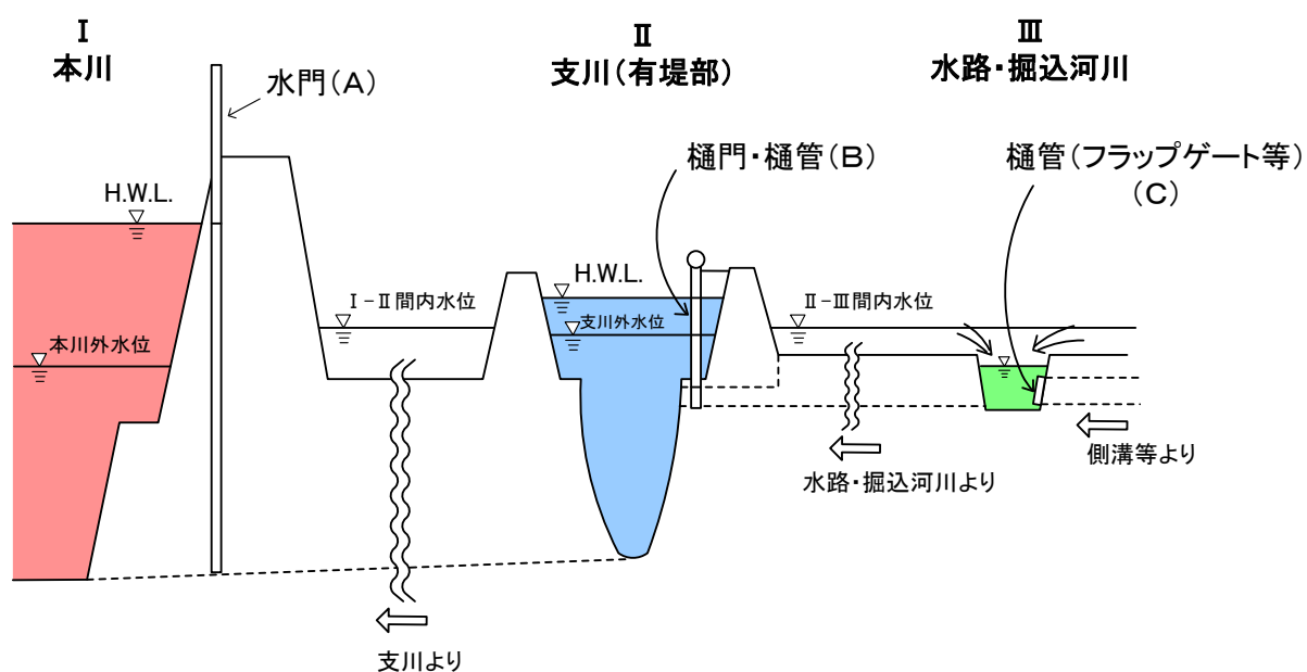
想定断面図
