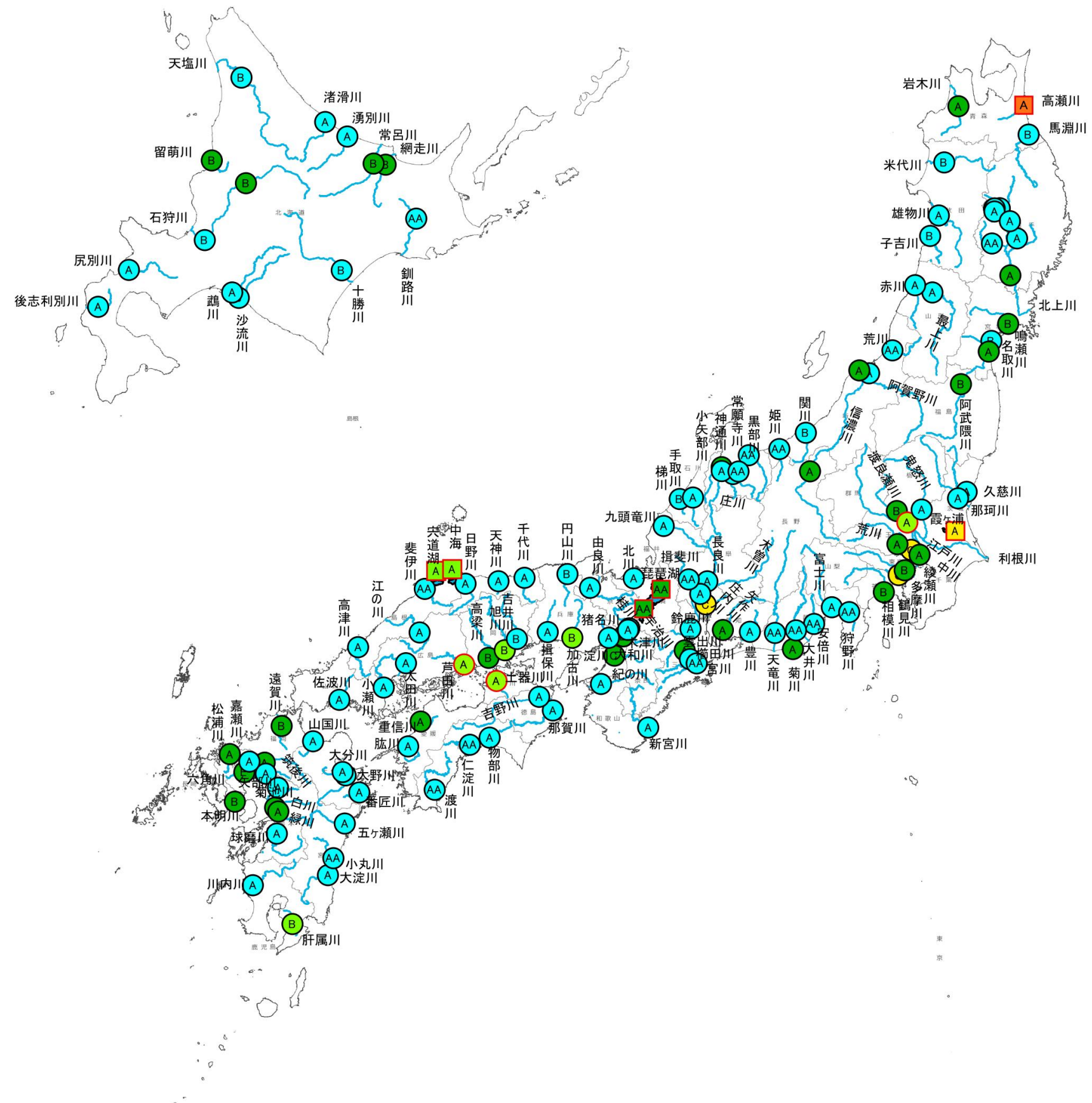
図-7 令和7年一級河川の水質状況図（主要地点のみ） （河川主要地点はBOD75値 湖沼主要地点はCOD75値）
