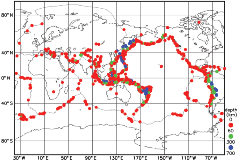
(注) 2012年～2021年 出典: アメリカ地質調査所の震源データより気象庁作成
