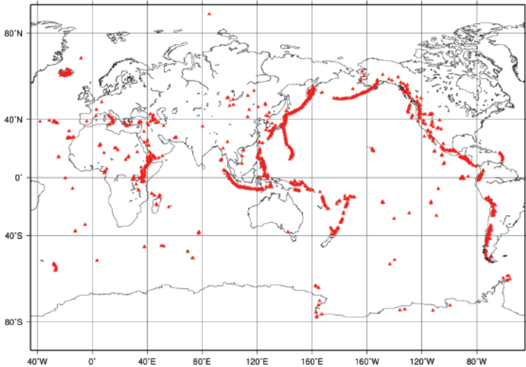
(注) 火山は過去概ね1万年間に活動のあったもの 出典: スミソニアン自然史博物館(アメリカ)のGrobal Volcanism Programによる火山データをもとに、気象庁作成
