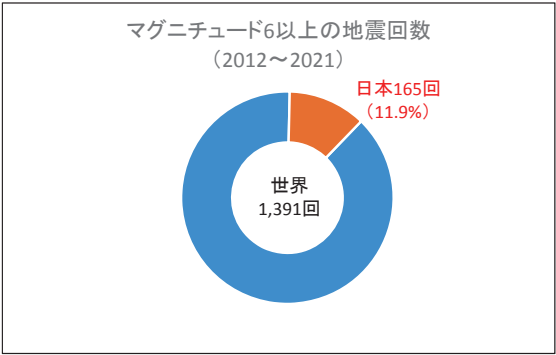
出典: アメリカ地質調査所(世界) 気象庁(日本)
