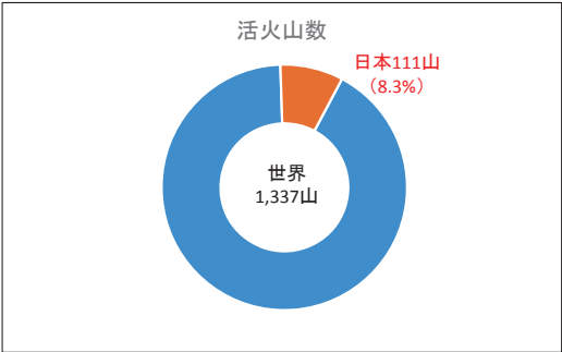
出典: スミソニアン自然史博物館(世界) 気象庁(日本)
