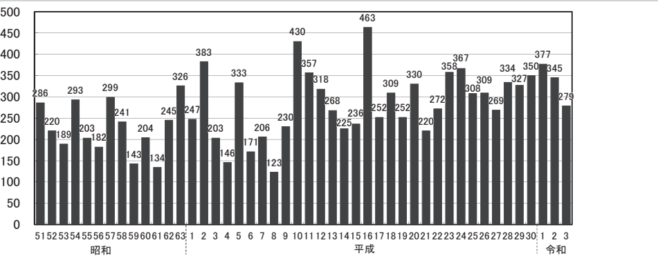
1時間降水量50mm以上の年間発生回数（アメダス1,300地点あたり）
