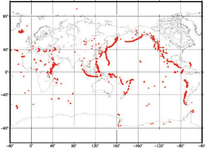
世界の火山の分布状況
