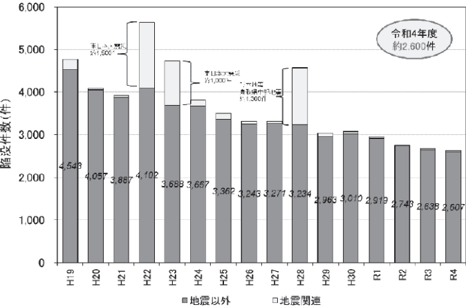
8-2-9 管路施設に起因する道路陥没件数の推移 (令和4年度末)
