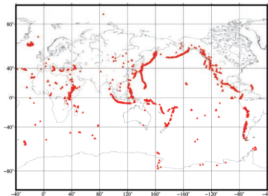
世界の火山の分布状況
