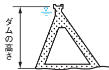
中空重力式コンクリートダム
