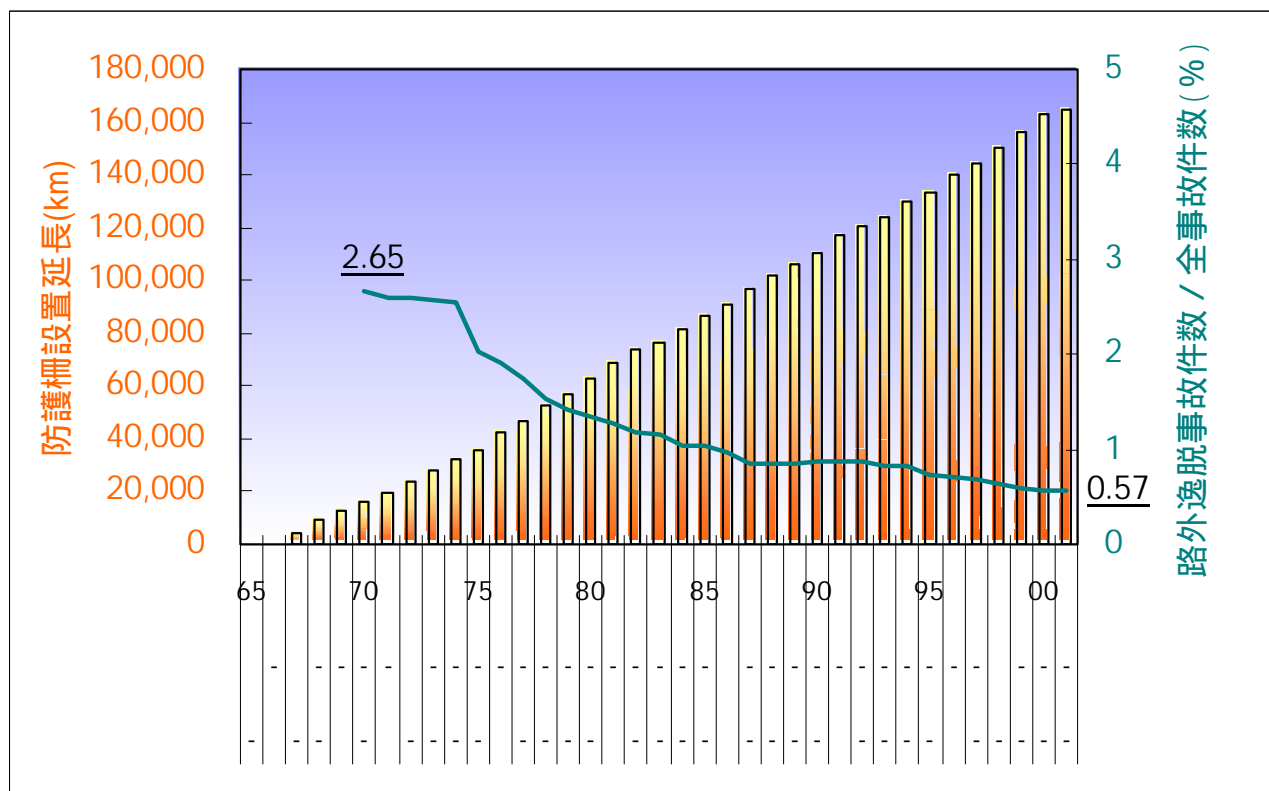
《防護柵設置延長と路外逸脱事故件数 / 全事故件数(%)の推移》
