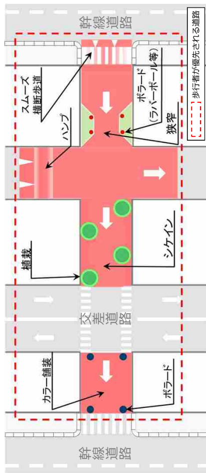
進入・速度抑制対策イメージ
