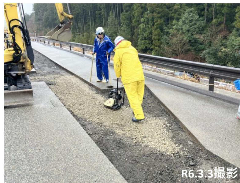
No.44付近 路盤不陸整正転圧状況
