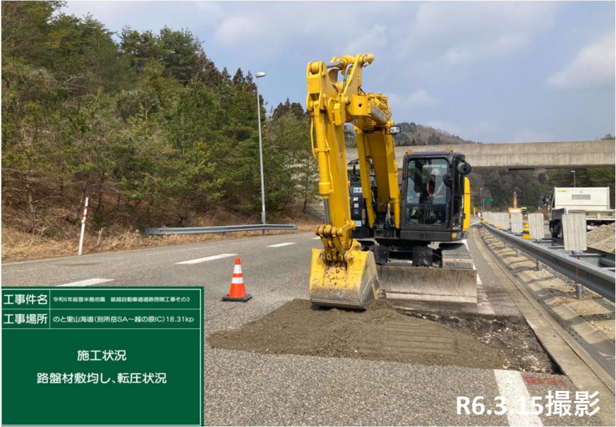
No.5路盤材敷均し、転圧状況
