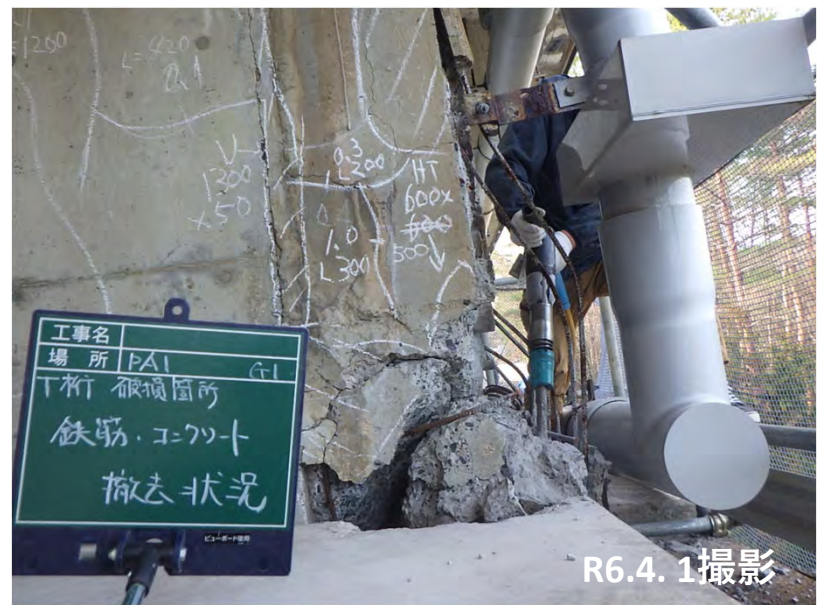
能登大橋・PA1橋台 鉄筋・コンクリート撤去状況
