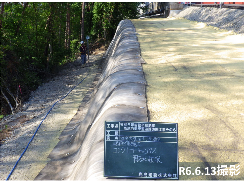
No.50 法面保護工状況
