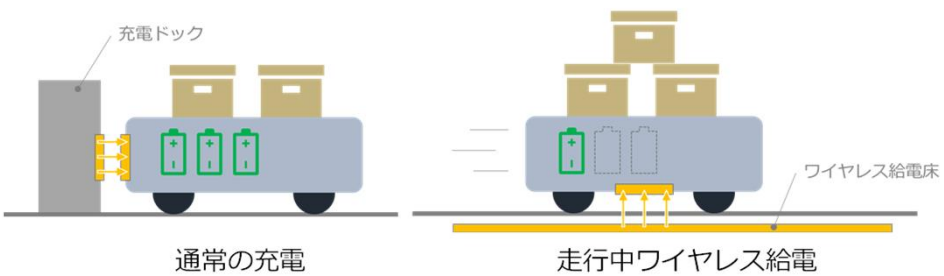
図1-3 走行中無線給電によるバッテリー削減効果のイメージ
