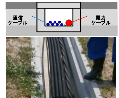
《小型ボックス活用埋設》
