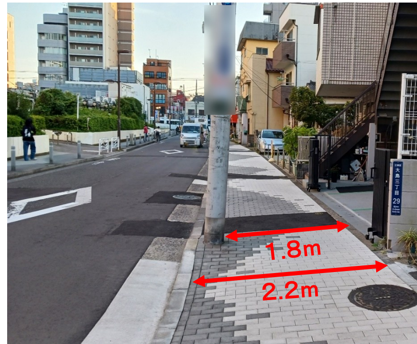
【電柱撤去により幅員2.0m以上を確保できる事例】
