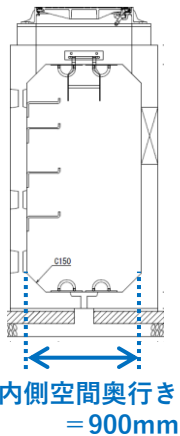
電線共同溝整備マニュアルに準じた分岐柵
