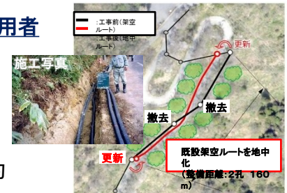
電力レジリエンス強化を目的に、更新に合わせた単独地中化の事例
