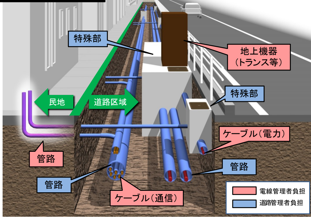
電線共同溝(管路直接埋設)
