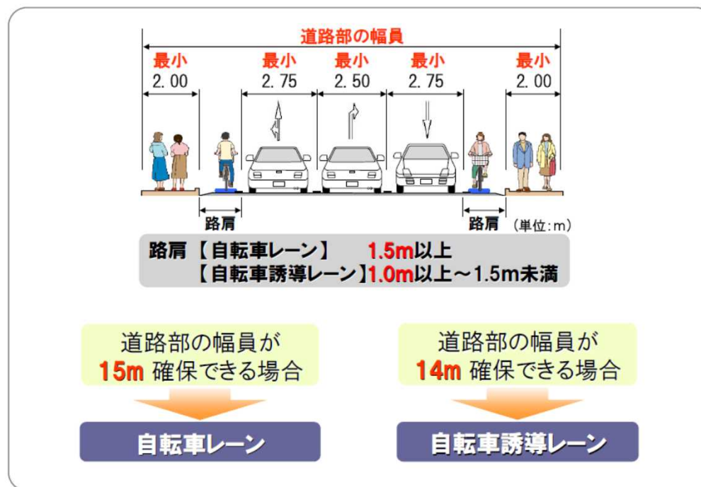
図- 5.17 道路空間の再配分 算定例
