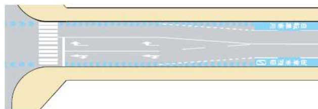
③自転車専用通行帯を打ち切り、進行方向を示す法定外表示を設置（当面の措置）
