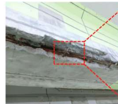
桁の変状状況
