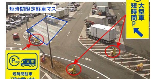
看板等設置状況 （古賀SA(下り)）
