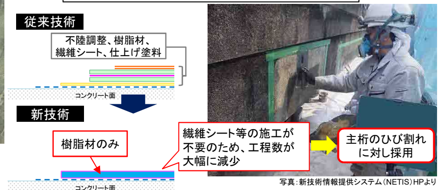
主桁のひび割れ
