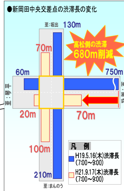
●渋滞状況の変化 [新岡田中央 intersection (綾歌工区)]
