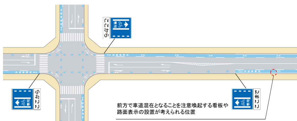
図Ⅱ-51 混在の場合の車道混在を注意喚起する看板・路面表示の位置の例 (交差点流出側に自転車専用通行帯を確保可能な場合)
