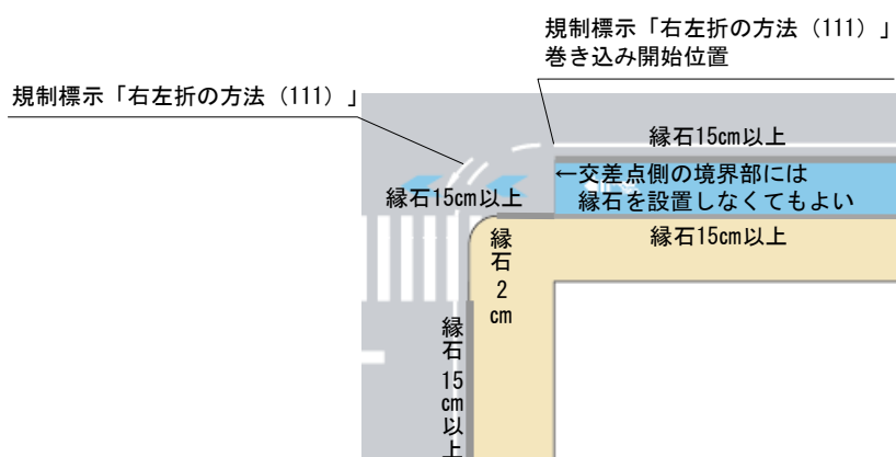
図Ⅱ-70 分離の場合の交差点隅角部の道路構造の例（従道路に歩道がある場合）
