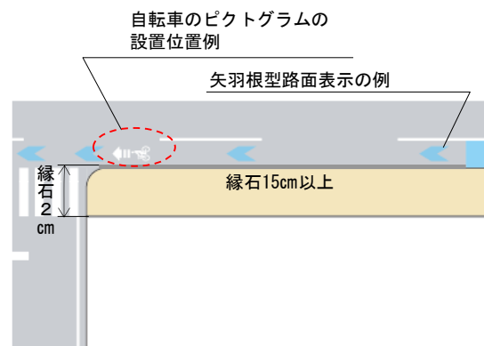
図Ⅱ-73 左折自動車のみ混在の場合の 交差点隅角部の道路構造の例 (自転車専用通行帯の場合)
