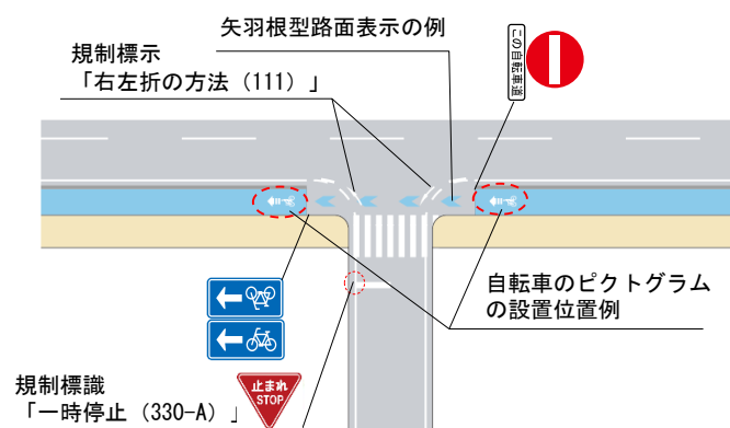
図Ⅱ-68 分離の場合の交差点イメージ （自転車道（自転車一方通行）の場合）
