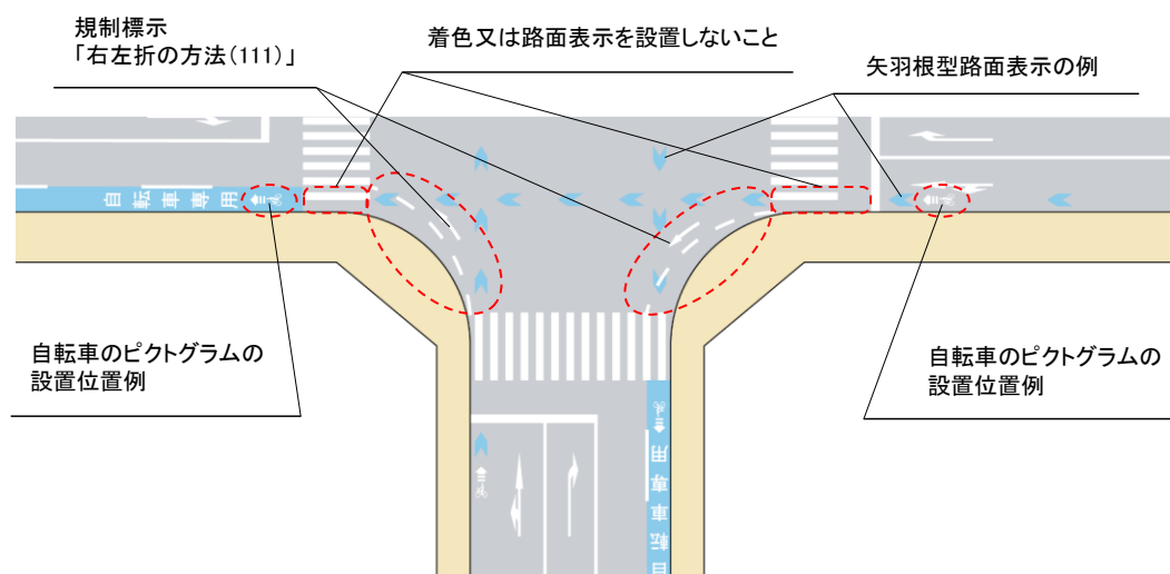
図Ⅱ-50 混在の場合の交差点隅角部の道路構造の例（自転車専用通行帯の場合）
