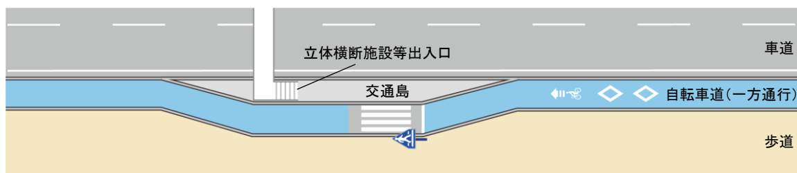
図Ⅱ-35 歩道空間を縮小して自転車道を設置する例（島型）
