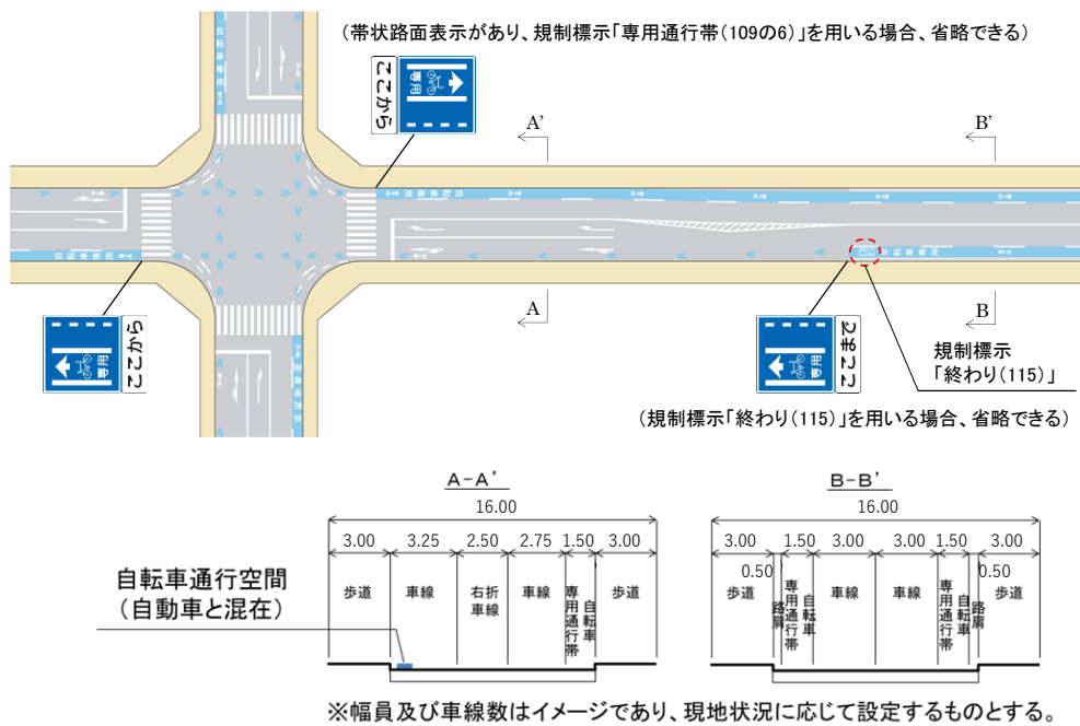
図Ⅱ-64 混在の場合の自転車専用通行帯が交差する交差点の例
