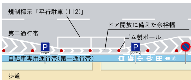
図Ⅱ-41 自転車専用通行帯の右側に駐車スペースを設置する例
