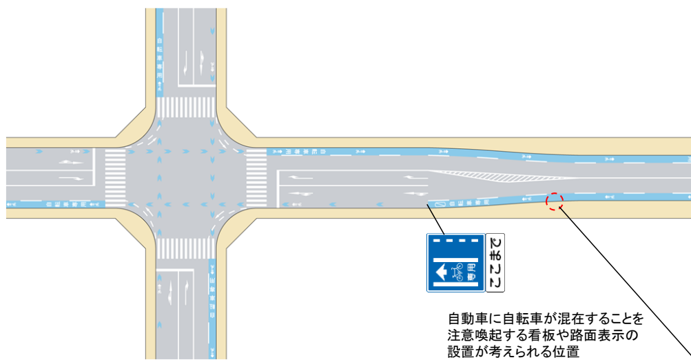
図Ⅱ-45 左折自動車のみ混在の場合の車道混在を注意喚起する看板・路面表示の位置の例（自転車専用通行帯の場合）
