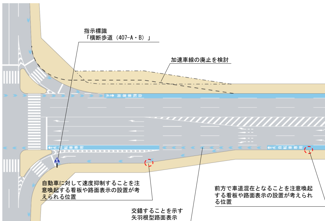
図Ⅱ-78 分離帯による導流路がある交差点の例 （自転車専用通行帯の場合）
