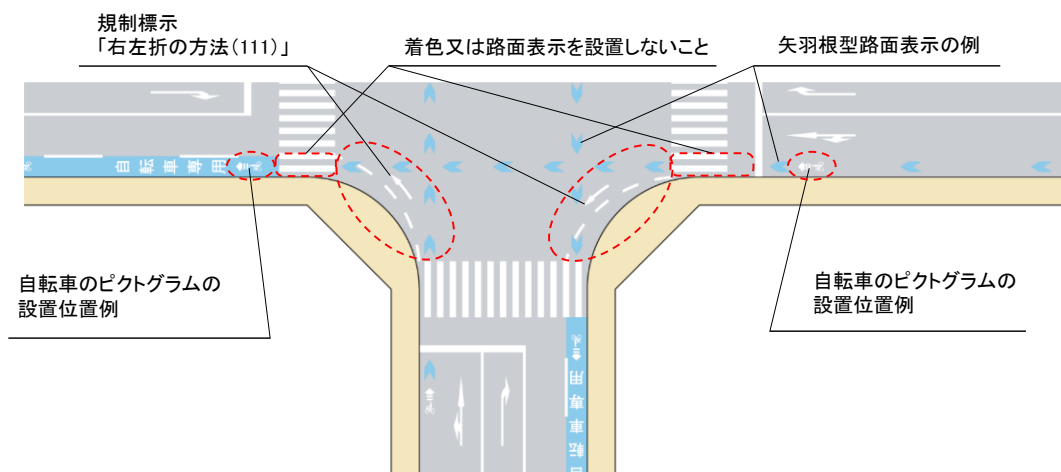
図Ⅱ-43 左折自動車のみ混在の場合の交差点隅角部の道路構造の例 (自転車専用通行帯の場合)
