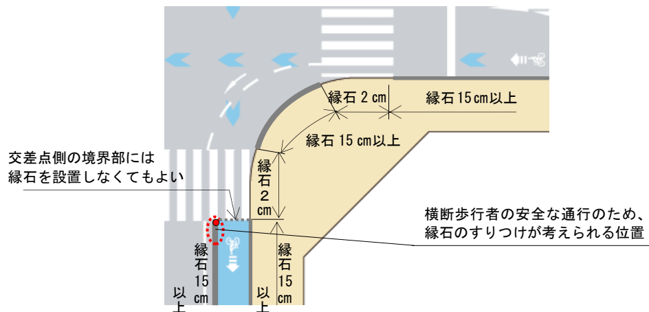
図Ⅱ-55 左折自動車のみ混在の場合の交差点隅角部の縁石構造の例 （自転車道（自転車一方通行）の場合）
