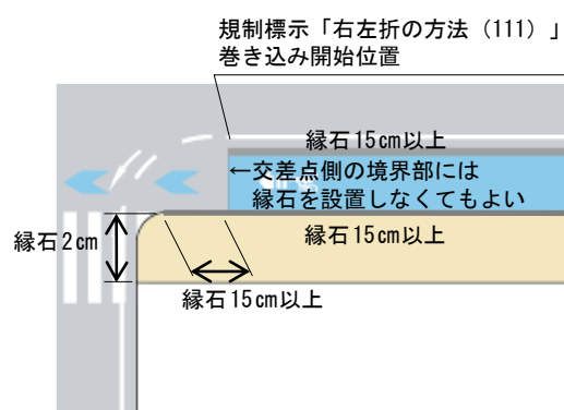
図Ⅱ-69 分離の場合の交差点隅角部の 道路構造の例 （自転車道（自転車一方通行）の場合）
