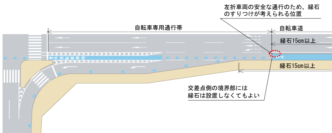
図Ⅱ-79 自転車道における分流部の縁石構造の例
