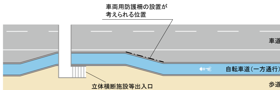
図Ⅱ-34 歩道空間を縮小して自転車道を設置する例（テラス型）
