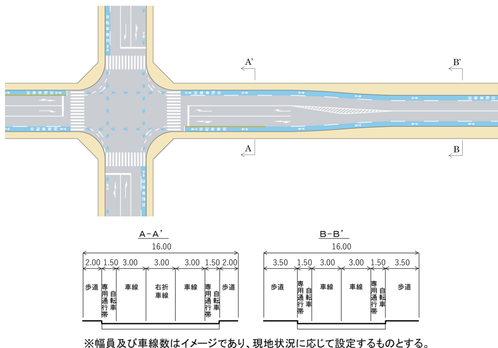
図Ⅱ-62 分離の場合の自転車専用通行帯が交差する交差点の例
