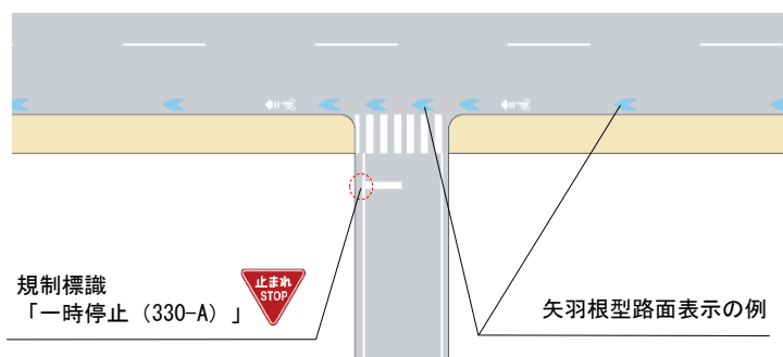
図Ⅱ-74 交差点イメージ（車道混在の場合）
