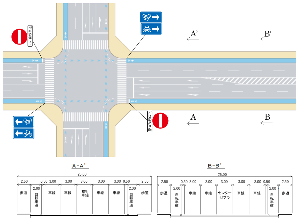
図Ⅱ-57 分離の場合の自転車道（自転車一方通行）が交差する交差点の例
