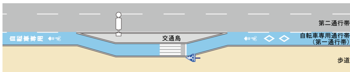
図Ⅱ-32 交通島を設置する例
