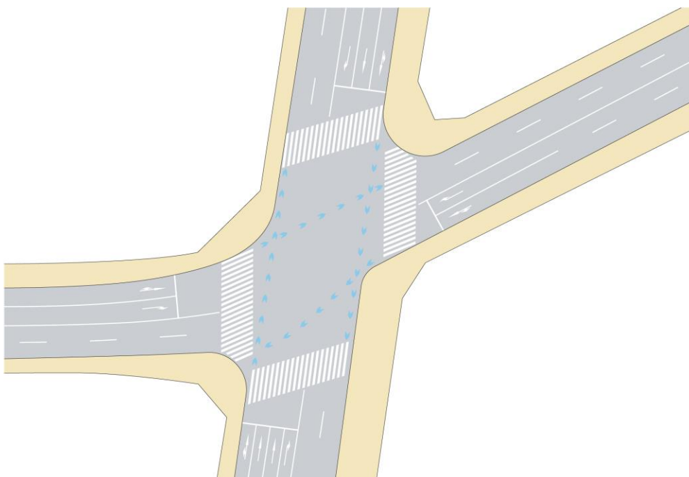
図Ⅱ-82 くい違い交差点における矢羽根型路面表示の設置例
