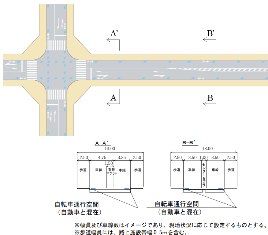
図Ⅱ-66 車道混在が交差する交差点の例
