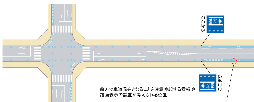
図Ⅱ-52 混在の場合の車道混在を注意喚起する看板・路面表示の位置の例 (交差点流出側に自転車専用通行帯を確保できない場合)
