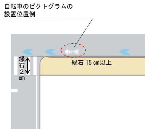
図Ⅱ-75 交差点隅角部の道路構造の例（車道混在の場合）
