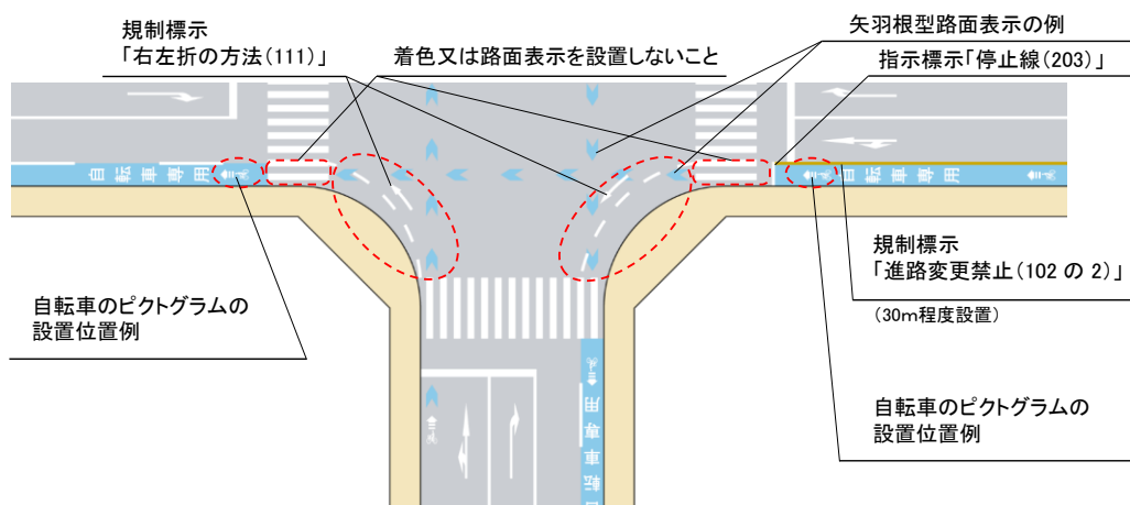
図Ⅱ-63 分離の場合の交差点隅角部の道路構造の例 (自転車専用通行帯の場合)
