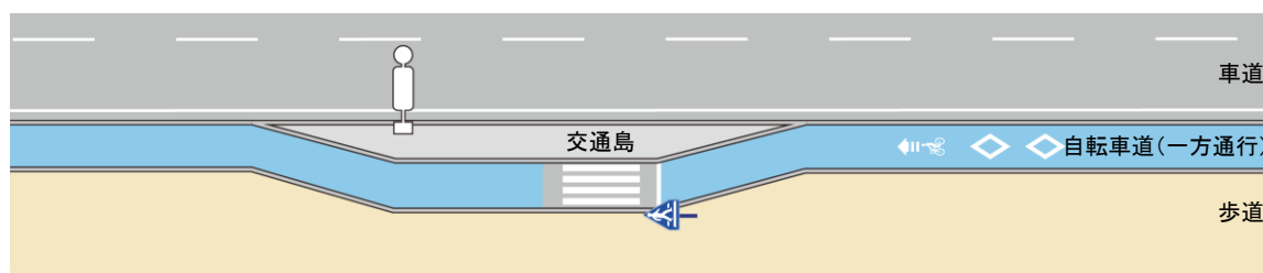
図Ⅱ-26 車道と自転車道との間に交通島のバス停留所を設ける例（島型） （バス交通が多く道路空間に余裕がある路線）
