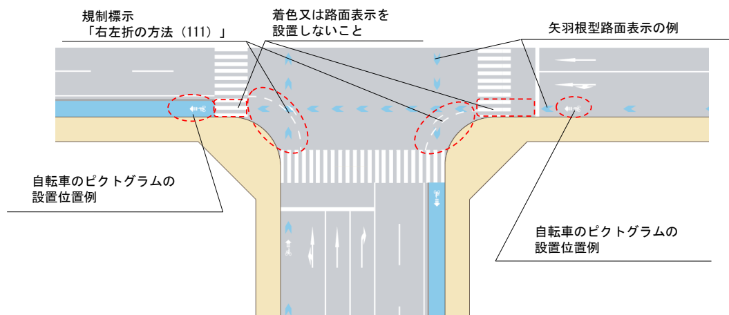
図Ⅱ-54 左折自動車のみ混在の場合の交差点隅角部の道路構造の例（自転車道（自転車一方通行）の場合）
