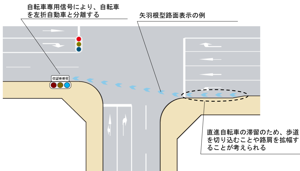
図Ⅱ-80 左折導流路のない左折可の交通規制が実施されている交差点の見直し例
