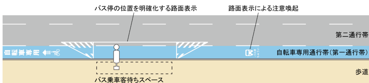
図Ⅱ-30 ストレート型バス停を設置する例
