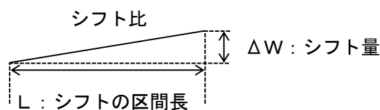
図Ⅱ-11 自転車道の屈曲部のシフト比
