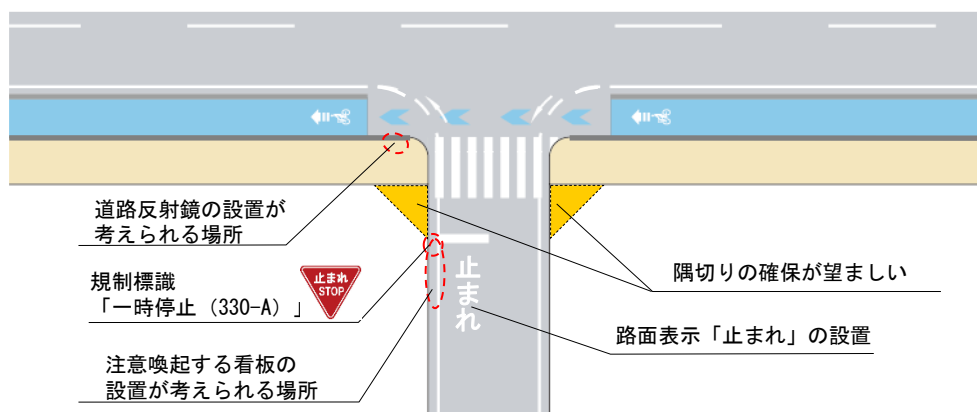
図Ⅱ-71 細街路側の道路構造の例
