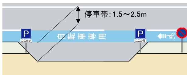
図Ⅱ-39 自転車専用通行帯の左側に停車帯を設置する例
