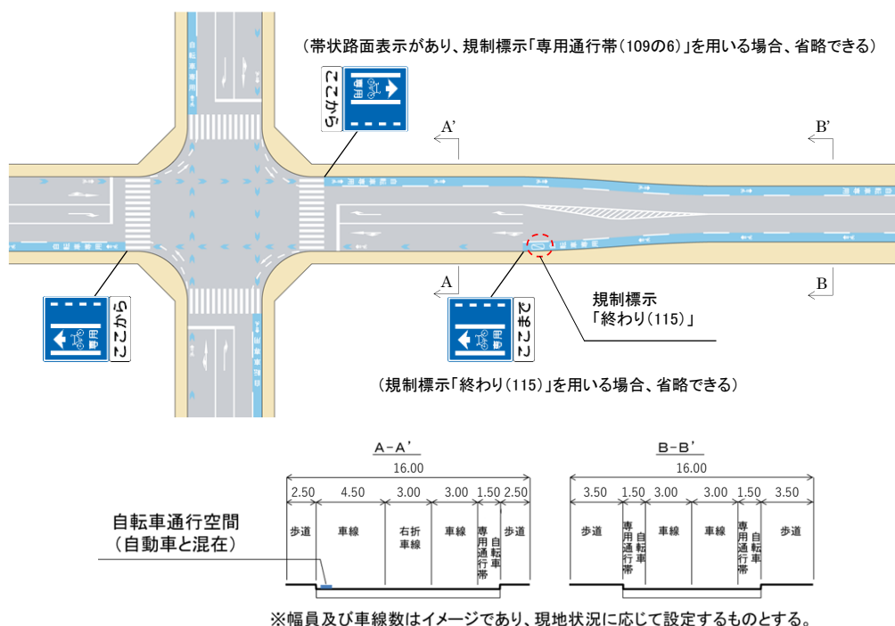
図Ⅱ-60 左折自動車のみ混在の場合の自転車専用通行帯が交差する交差点の例
