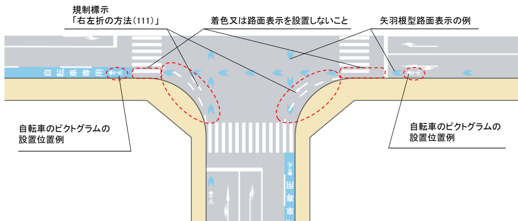
図Ⅱ-65 混在の場合の交差点隅角部の道路構造の例 (自転車専用通行帯の場合)
