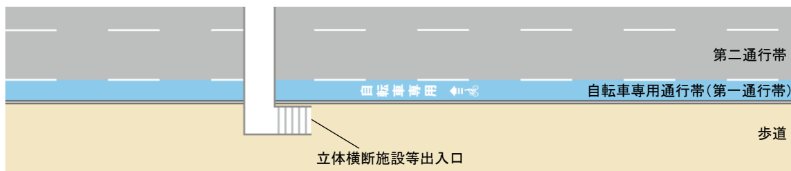
図Ⅱ-36 立体横断施設等出入口付近で自転車専用通行帯を設ける例
