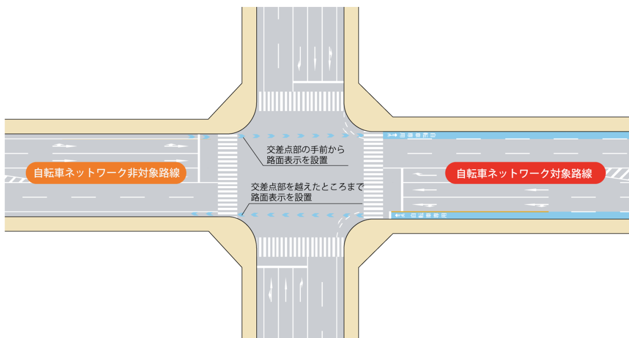
図Ⅱ-83 自転車ネットワーク端部の交差点部の路面表示方法の例
