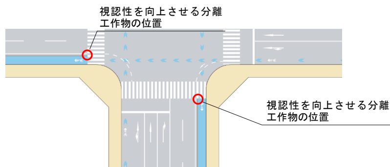
図Ⅱ-56 自転車道の分離工作物の視認性を向上させることが考えられる位置
