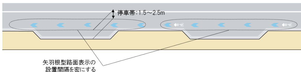
図Ⅱ-42 車道混在の道路に停車帯を設置する例
