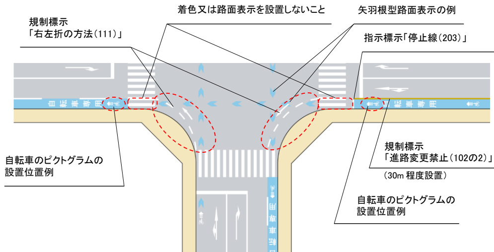
図Ⅱ-47 分離の場合の交差点隅角部の道路構造の例 (自転車専用通行帯の場合)
