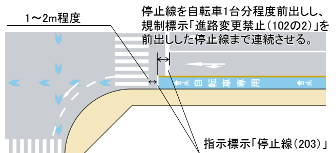
図Ⅱ-48 停止線の前出しの例 (自転車専用通行帯の場合)
