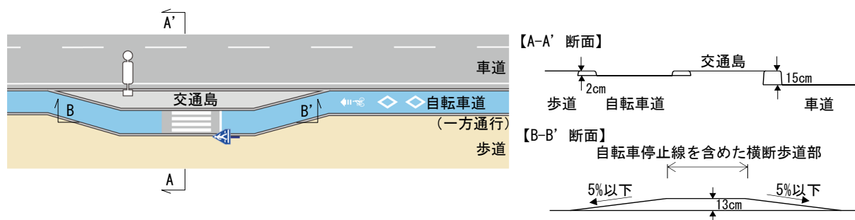
図Ⅱ-29 バス停部における高低差すりつけ方法の例
