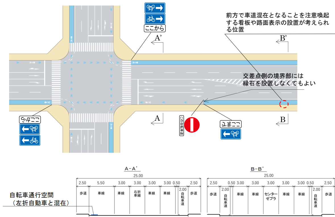
図Ⅱ-53 左折自動車のみ混在の場合の自転車道（自転車一方通行）が交差する交差点の例
