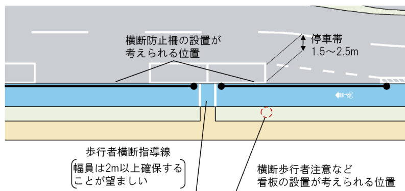
図Ⅱ-38 自転車道のある道路に停車帯を設置する例
