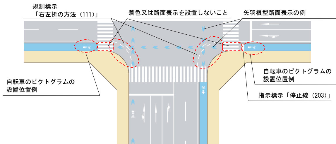
図Ⅱ-58 分離の場合の交差点隅角部の道路構造の例 （自転車道（自転車一方通行）の場合）
