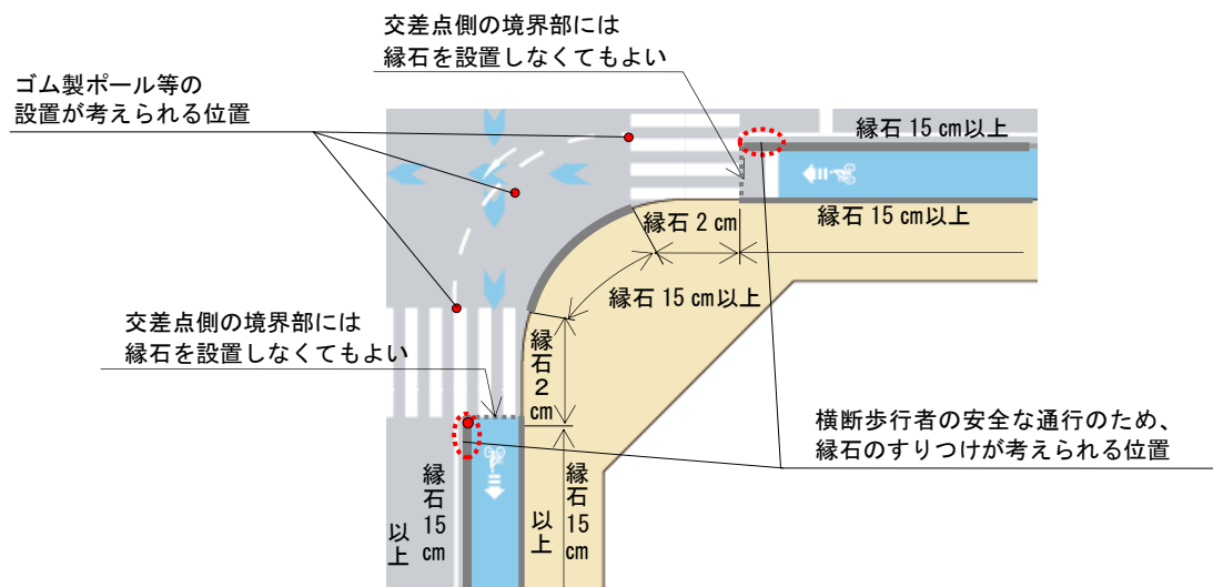
図Ⅱ-59 分離の場合の交差点隅角部の縁石構造の例 (自転車道(自転車一方通行)の場合)
