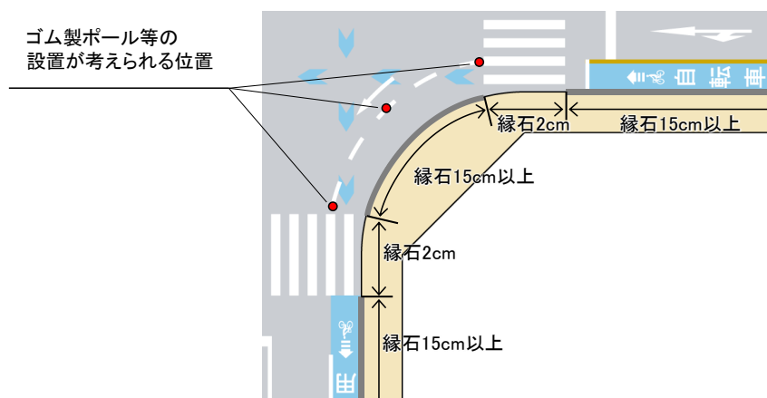
図Ⅱ-49 分離の場合の交差点隅角部の縁石構造の例（自転車専用通行帯の場合）
