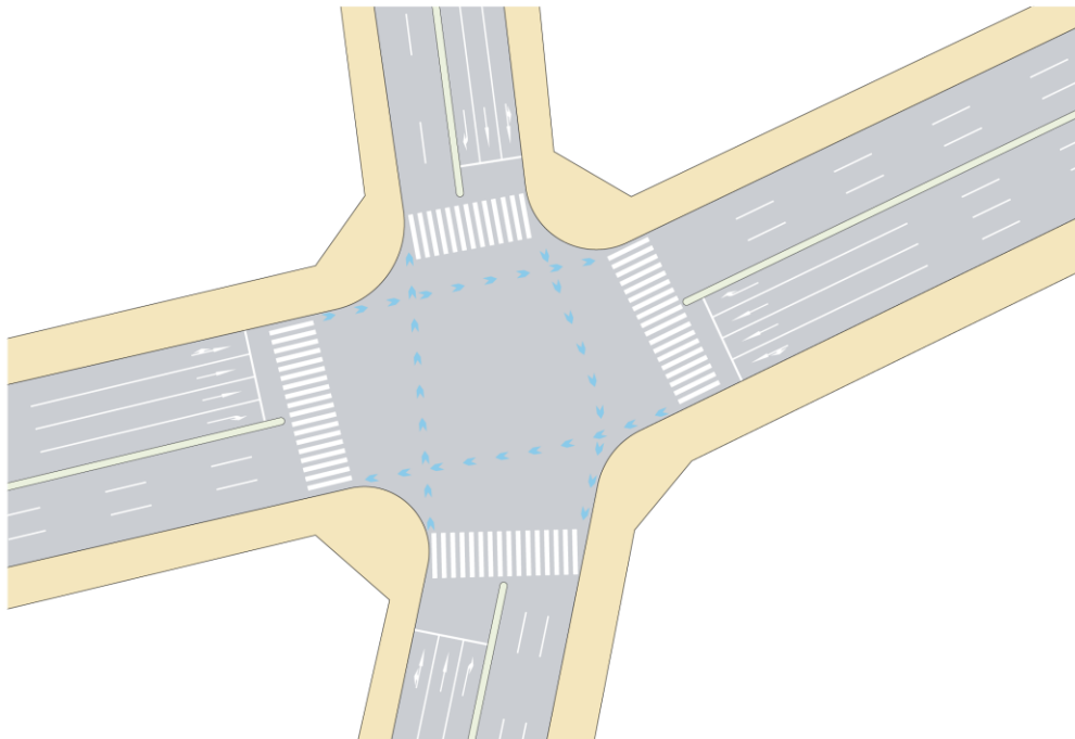
図Ⅱ-81 折れ脚交差点における矢羽根型路面表示の設置例
