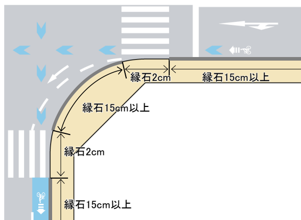
図Ⅱ-46 左折自動車のみ混在の場合の交差点隅角部の縁石構造の例（自転車専用通行帯の場合）
