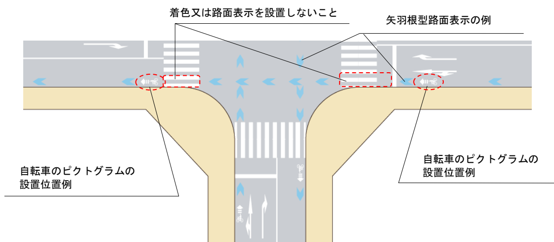
図Ⅱ-67 交差点隅角部の道路構造の例 (車道混在の場合)
