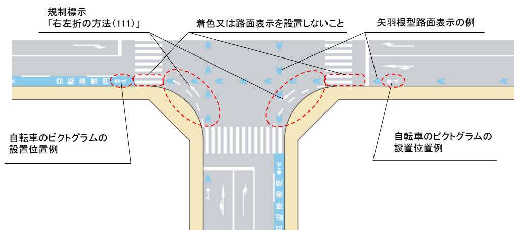
図Ⅱ-61 左折自動車のみ混在の場合の交差点隅角部の道路構造の例
