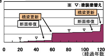
損傷がより深刻化してから対策を実施
