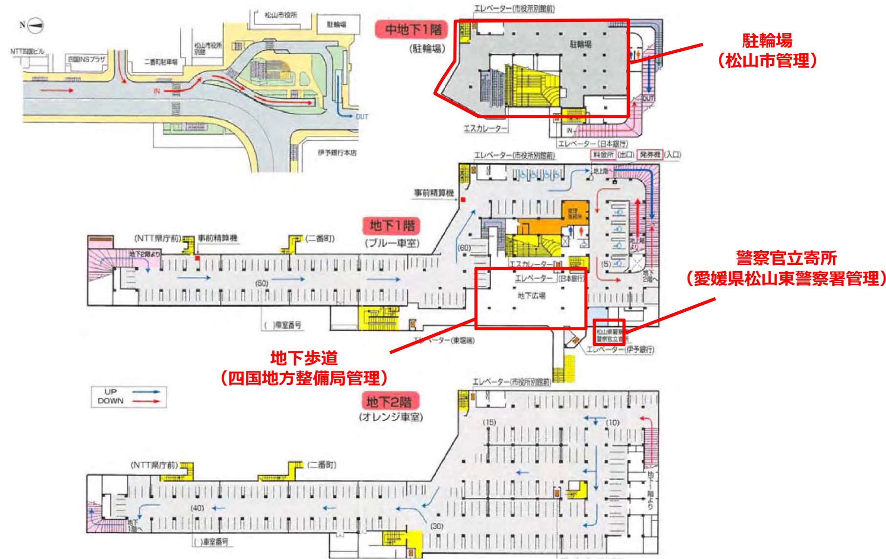
■ 概略配置図
