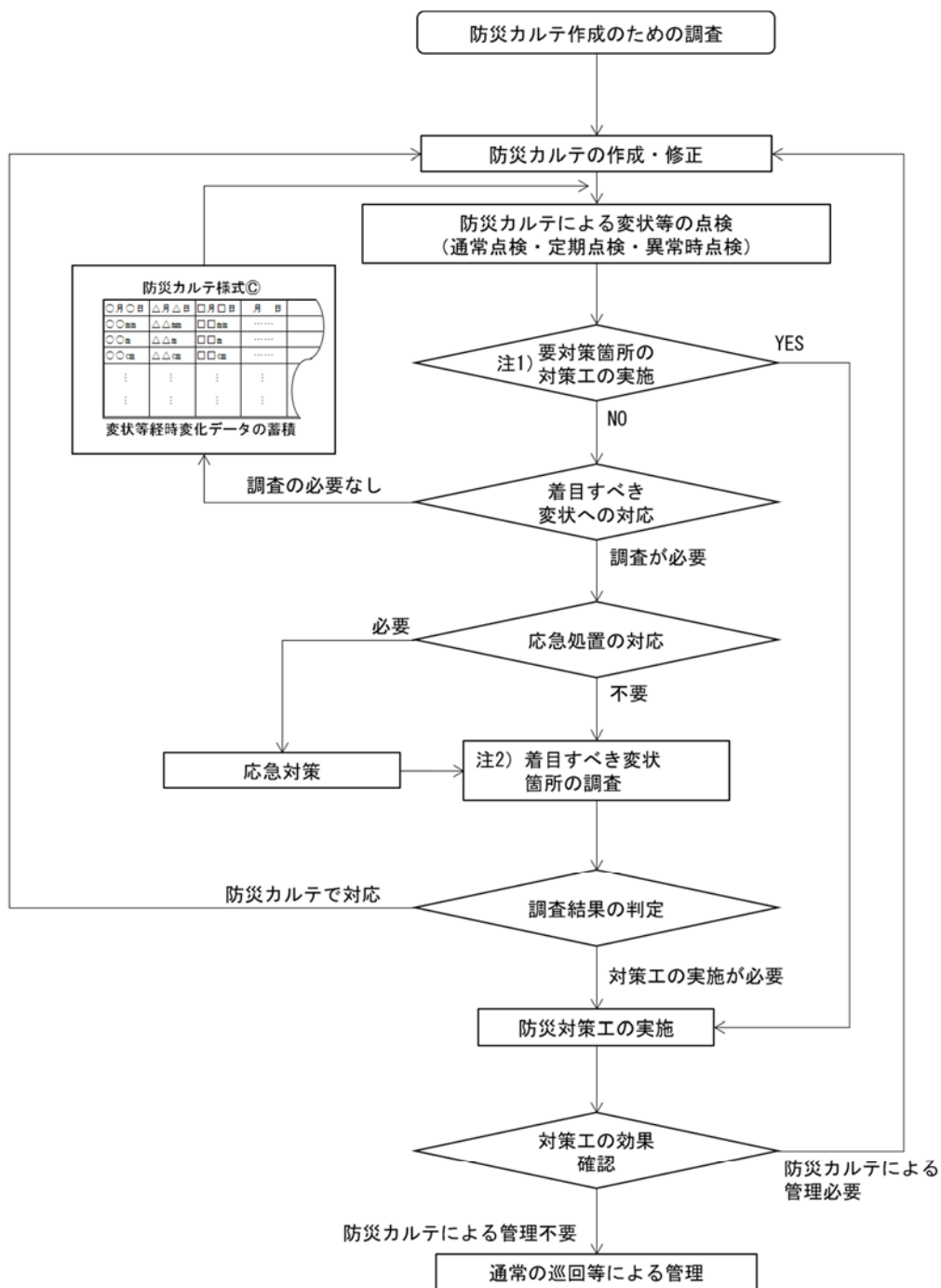
図-3-1 防災カルテを用いた点検・管理のフロー
