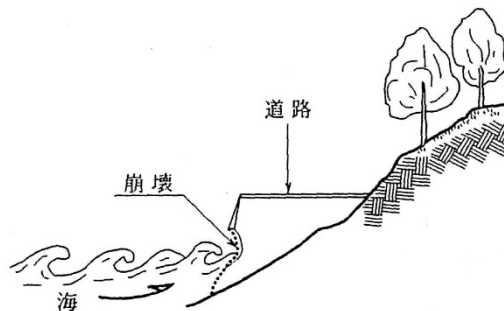
図-2-13(2) 波浪による浸食・崩壊
