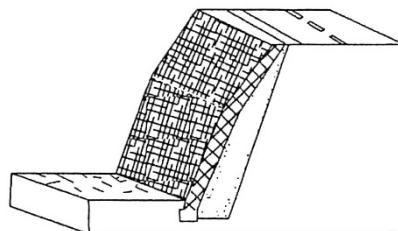
図-2-21 はらみだし
