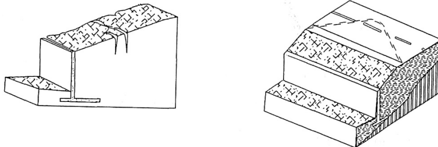
図-2-16 背面の亀裂
