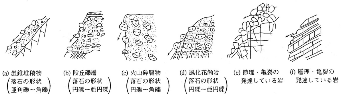
図-2-1 支持状態が不安定な浮石・転石の例
