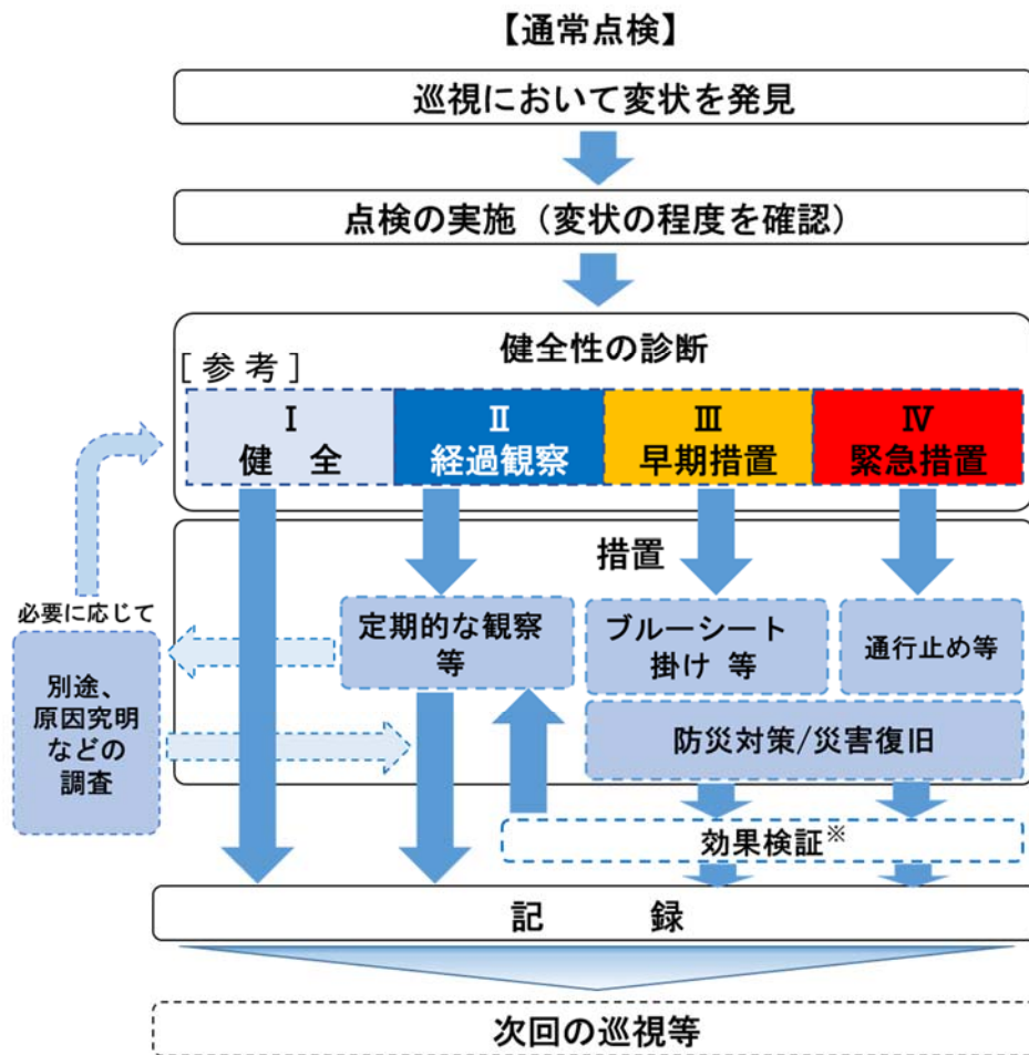
図-14 通常点検のフロー図
