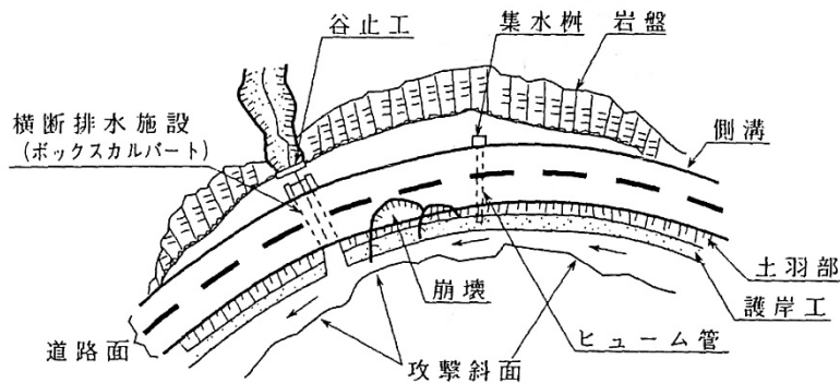
図-2-13(1) 河川の浸食による崩壊
