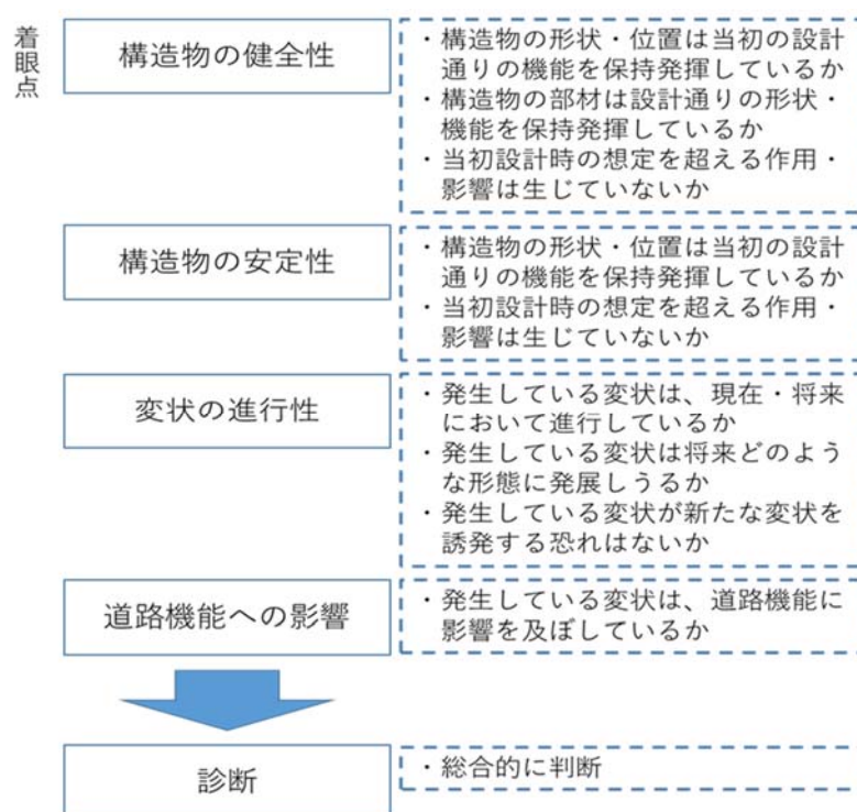
図-9 診断の着眼点
