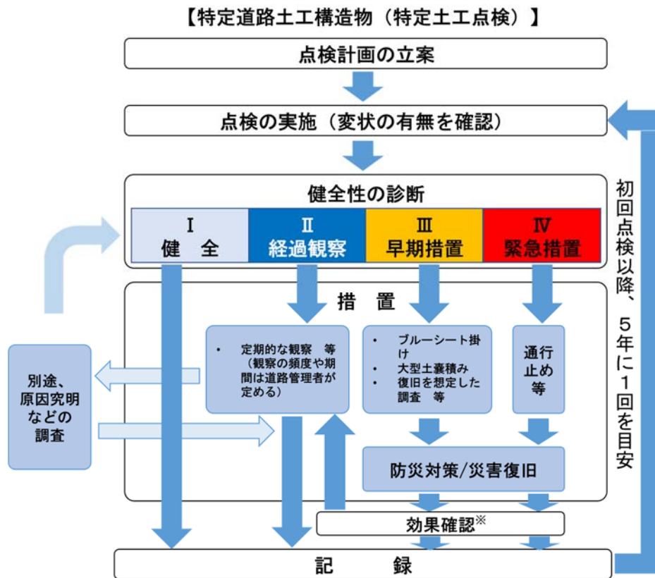
図-12 特定土工点検のフロー図
