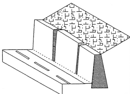
図-2-20 目地のずれ、段差
