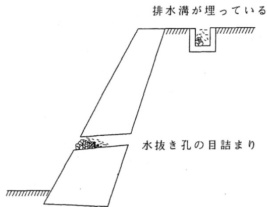
図-2-15 排水施設の機能低下
