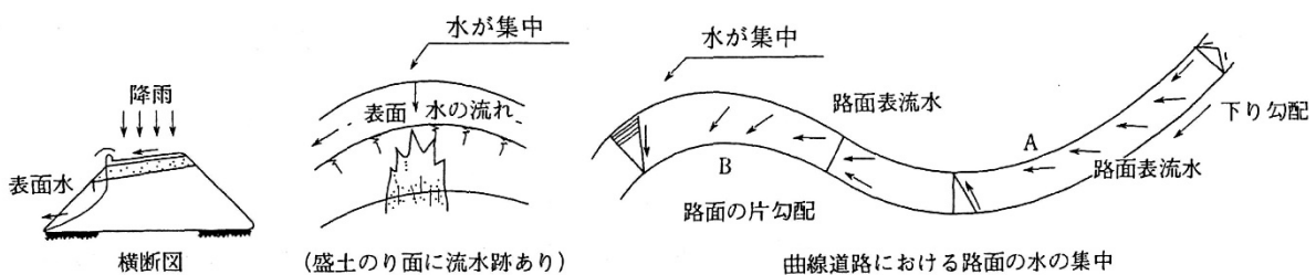
図-2-10 路面の水の集中とのり面の変状
