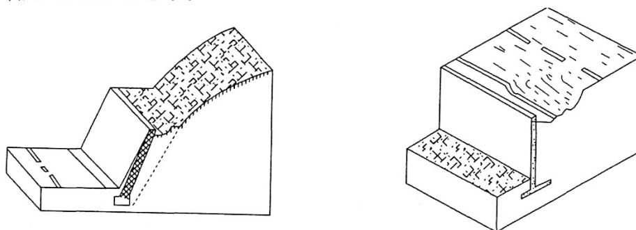
図-2-18 背面の陥没・沈下
