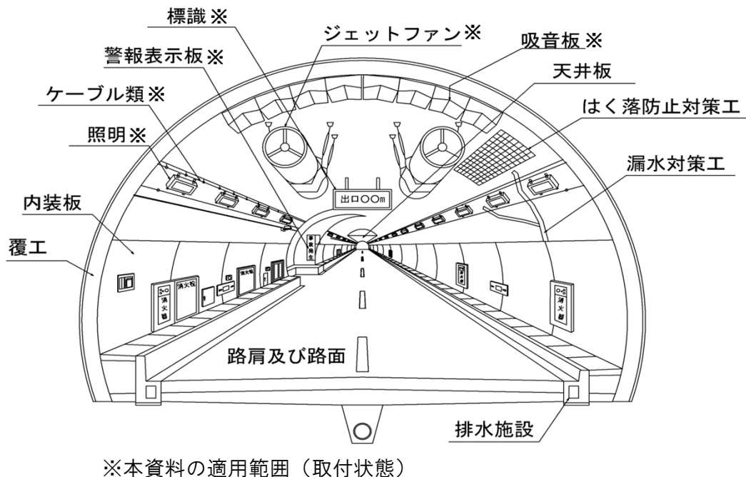
図-1 トンネル内附属物の取付状態等の確認の対象箇所
