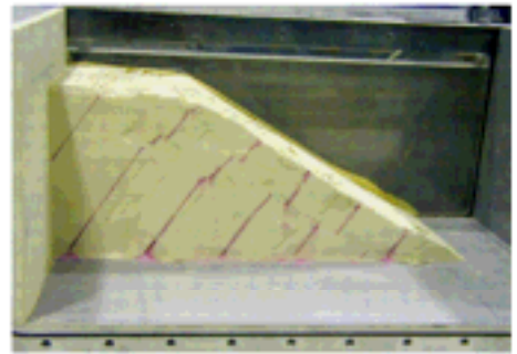
写真1 盛土のすべり破壊の遠心模型実験
