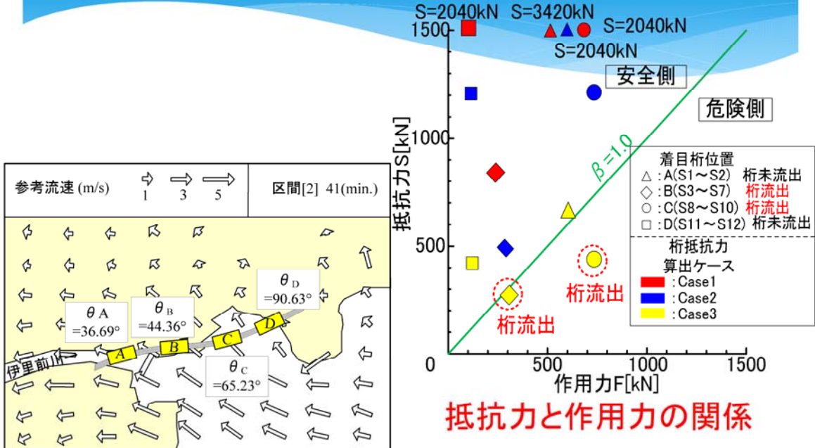
流速ベクトル図 (桁が完全に浸水した時点)
