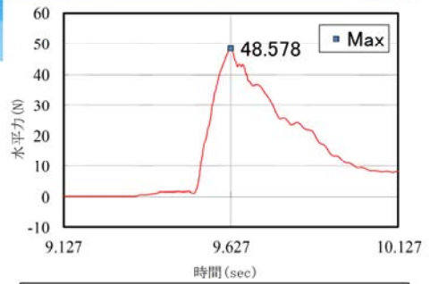
孤立波の水平波力 F_{x1}
