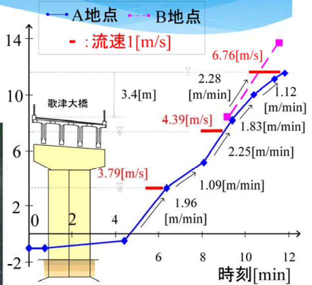
浸水高と流速の時刻歴変化
