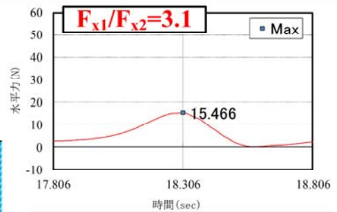
定常流＋孤立波の水平波力 F_{x2}
