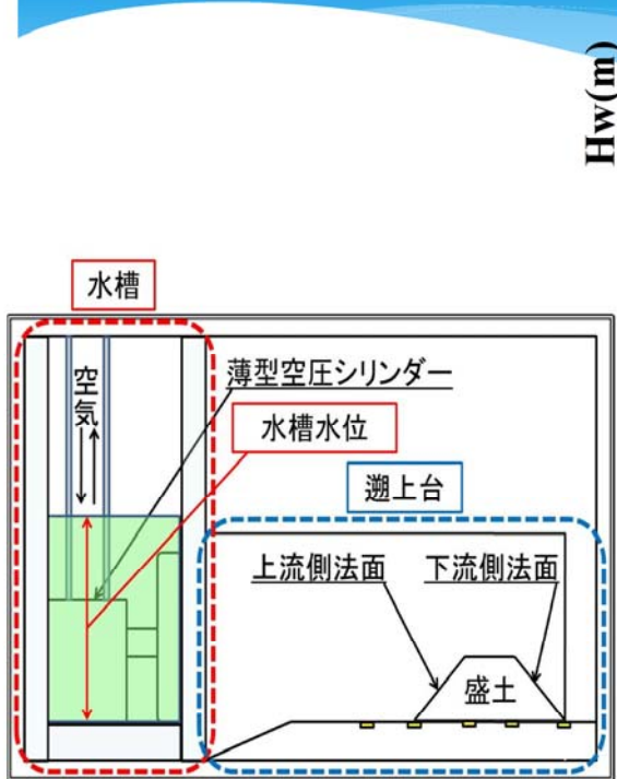
実験システム図
