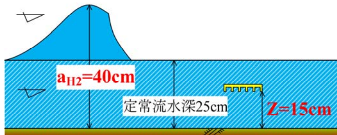
定常流＋孤立波の水平波力 F_{x2}
