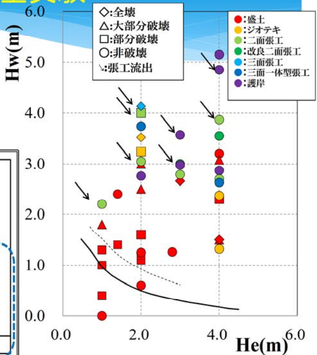
盛土高ー越流水深の関係
