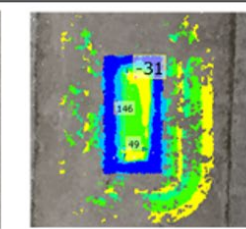
差分解析による求積
