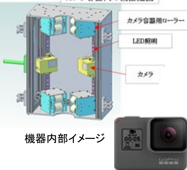
カメラ容器内の機器配置
