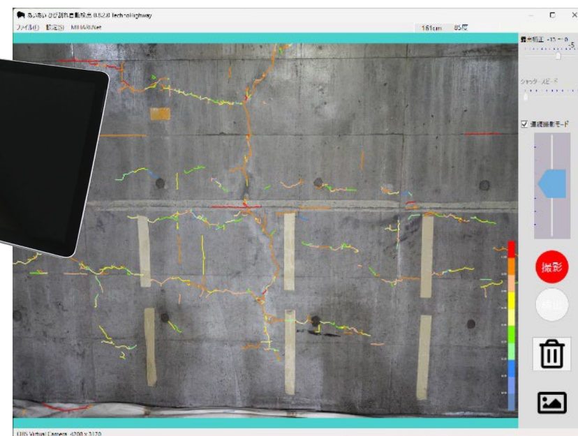
あいあい本体
