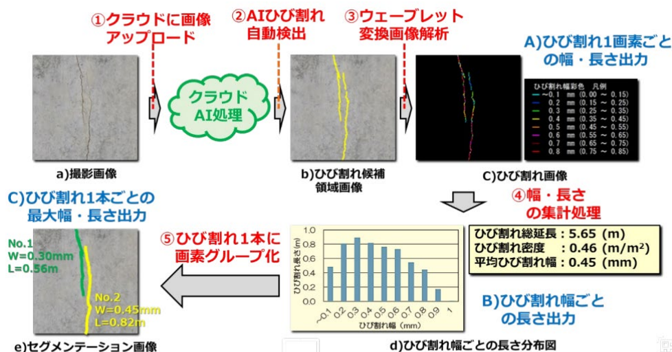
t.WAVEによるひび割れ画像解析の実施手順
