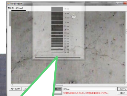
ひびわれ幅計測(画面上)
