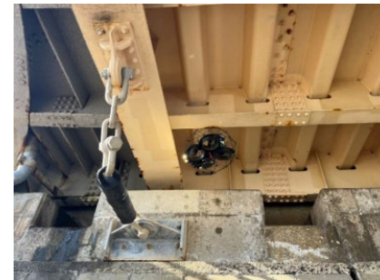
球体ガードで狭い箇所でも安心
