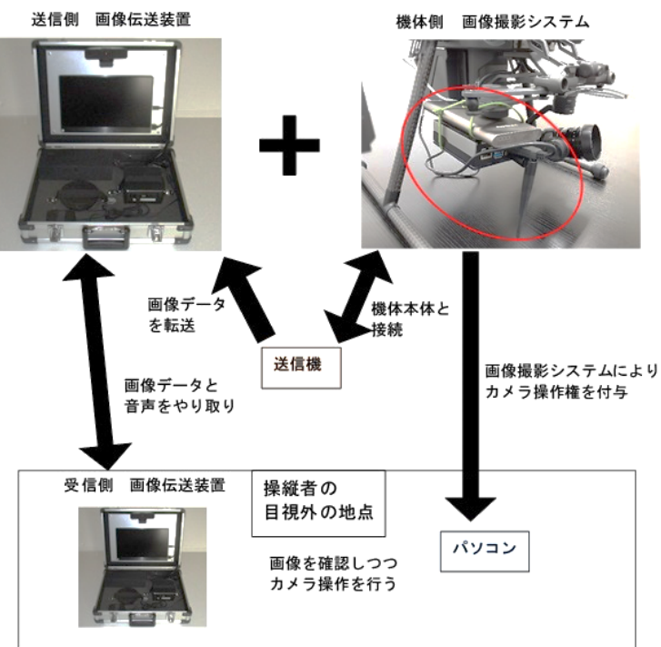
送信側 画像伝送装置
