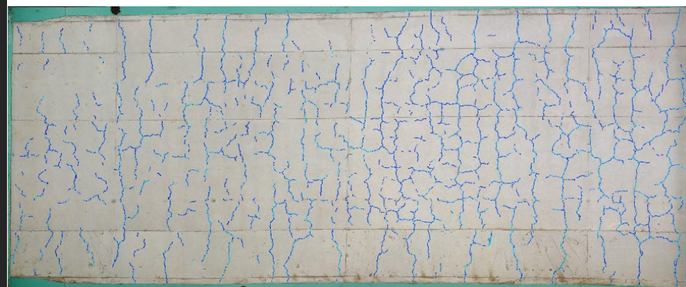
橋梁点検クラック分布図
