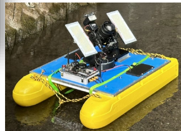
KENBOT-ASV 3号機
