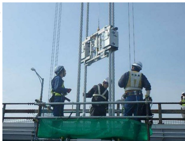
装置取付状況
