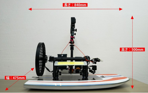
機体寸法
