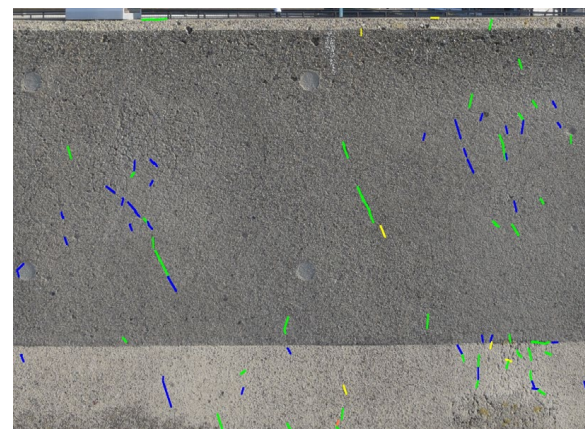
ひび検出結果画像
