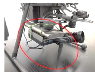
機体側 画像撮影システム
