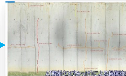
AI解析
