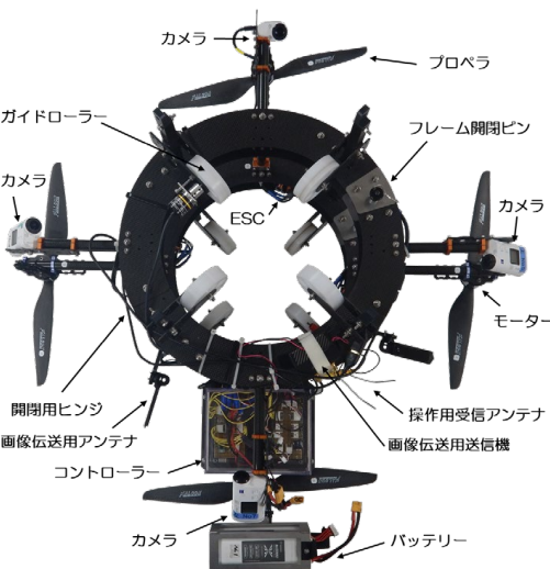
ロボットの構成
