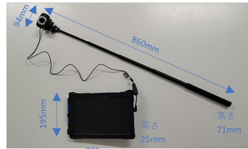
図2. 装置寸法
