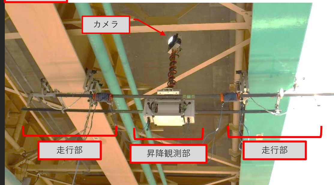
本体外観
