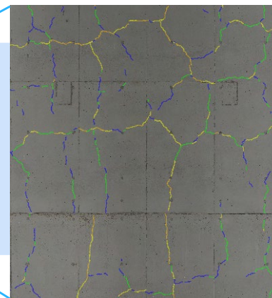
AIを用いたひびわれの自動検出
