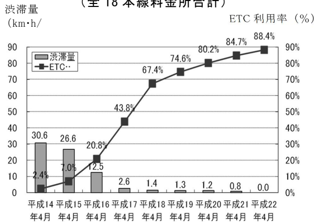
【ETC 利用率と本線料金所渋滞量の関係】 (全 18 本線料金所合計)
