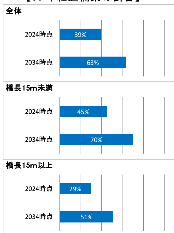
【50 年経過橋梁の割合】
