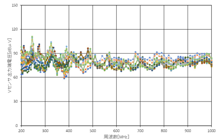
【RVC 法測定結果例】
