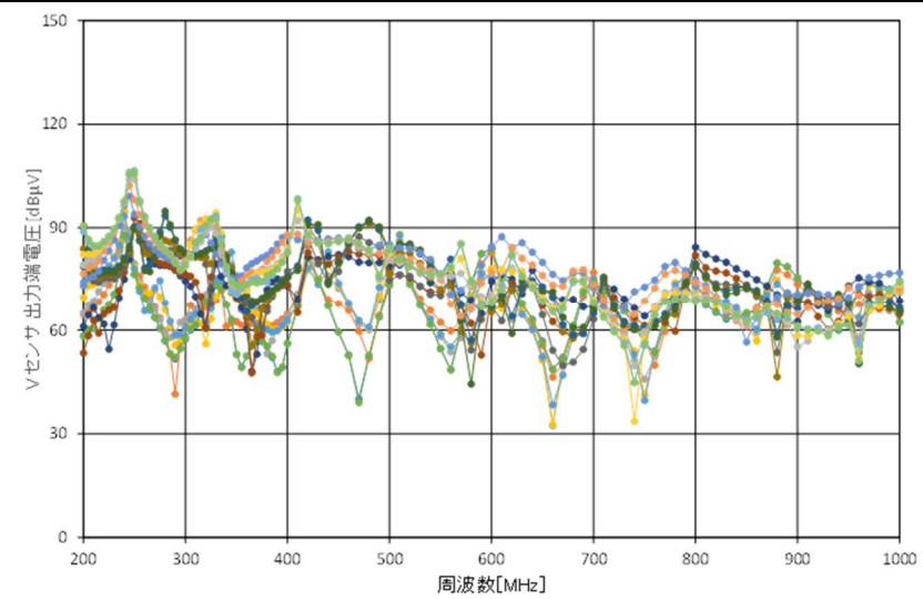
【ALSE 法測定結果例】
