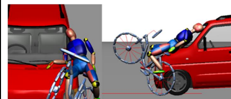
頭部とAピラーが衝突する場合
