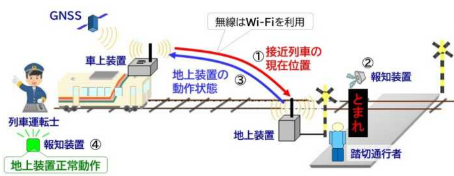
【図2 第4種踏切安全通行支援システムの概略】
