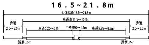
京都今出川線の道路断面
