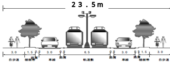
LRT導入時の標準的な横断面構成
