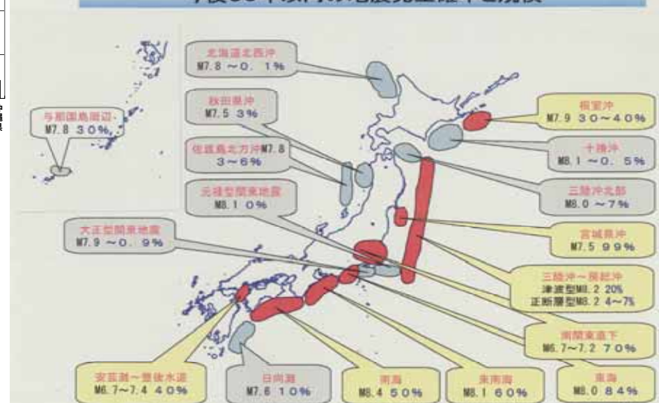
今後30年以内の地震発生確率と規模
