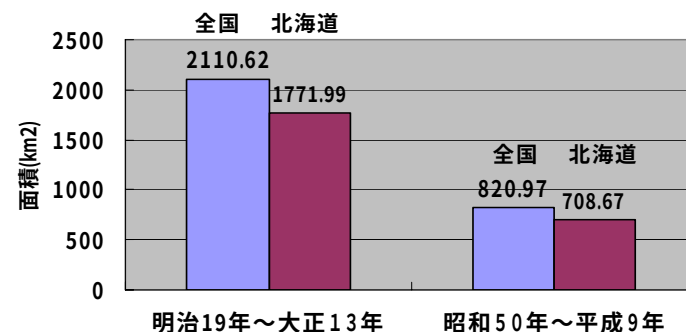
湿地面積の変化
