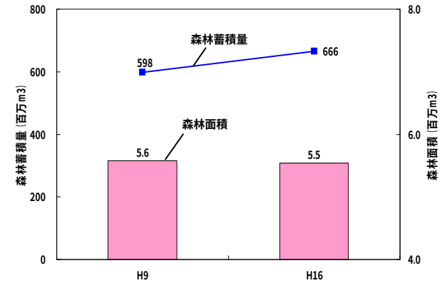
森林面積及び蓄積量の推移
