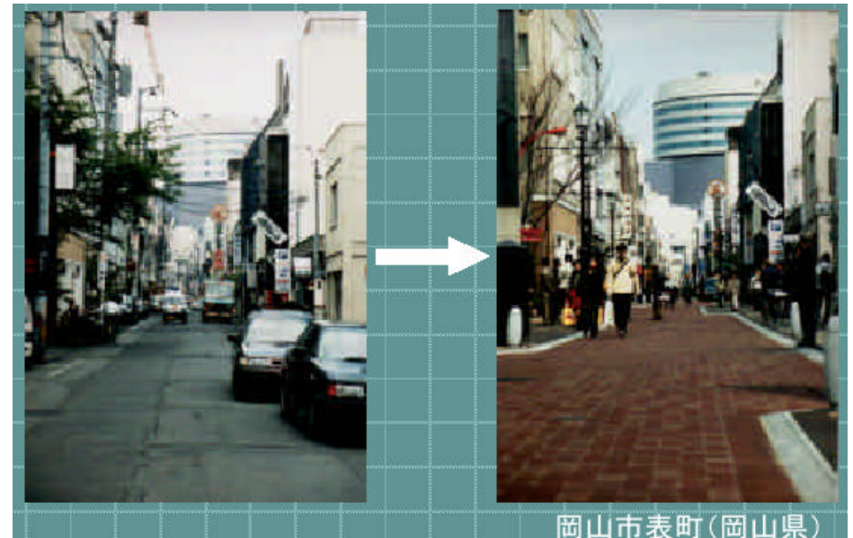
電線地中化施工例
