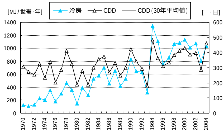
図、3、冷房度日と冷房用エネルギー消費量(住環境計画研究所推計)
