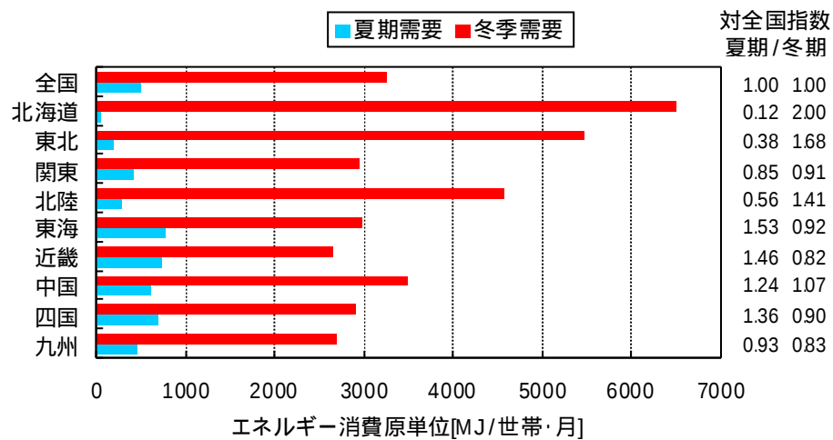
図、1、地域別夏期・冬季のエネルギー消費量の比較(住環境計画研究所推計)
