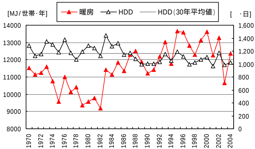
図、4、暖房度日と暖房用エネルギー消費量(住環境計画研究所推計)
