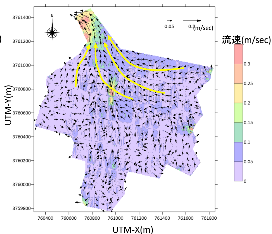
潮流流速分布・流速ベクトル (下げ潮時・水深平均)
