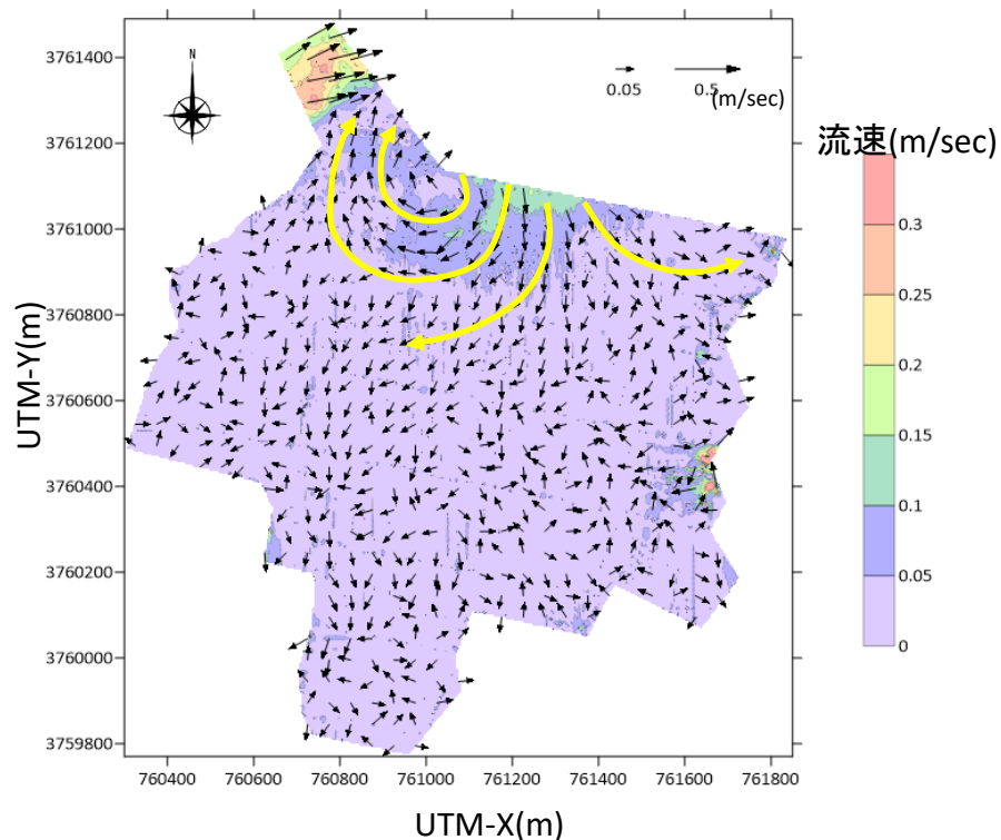
潮流流速分布・流速ベクトル (上げ潮時・水深平均)
