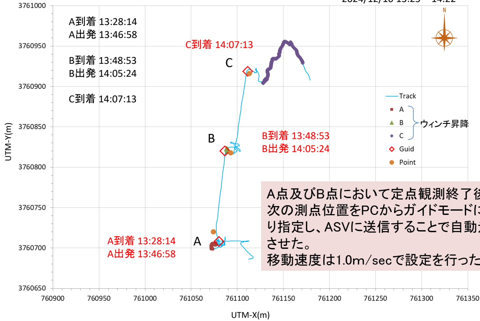
ASV定点観測時の航跡及び計測地点
