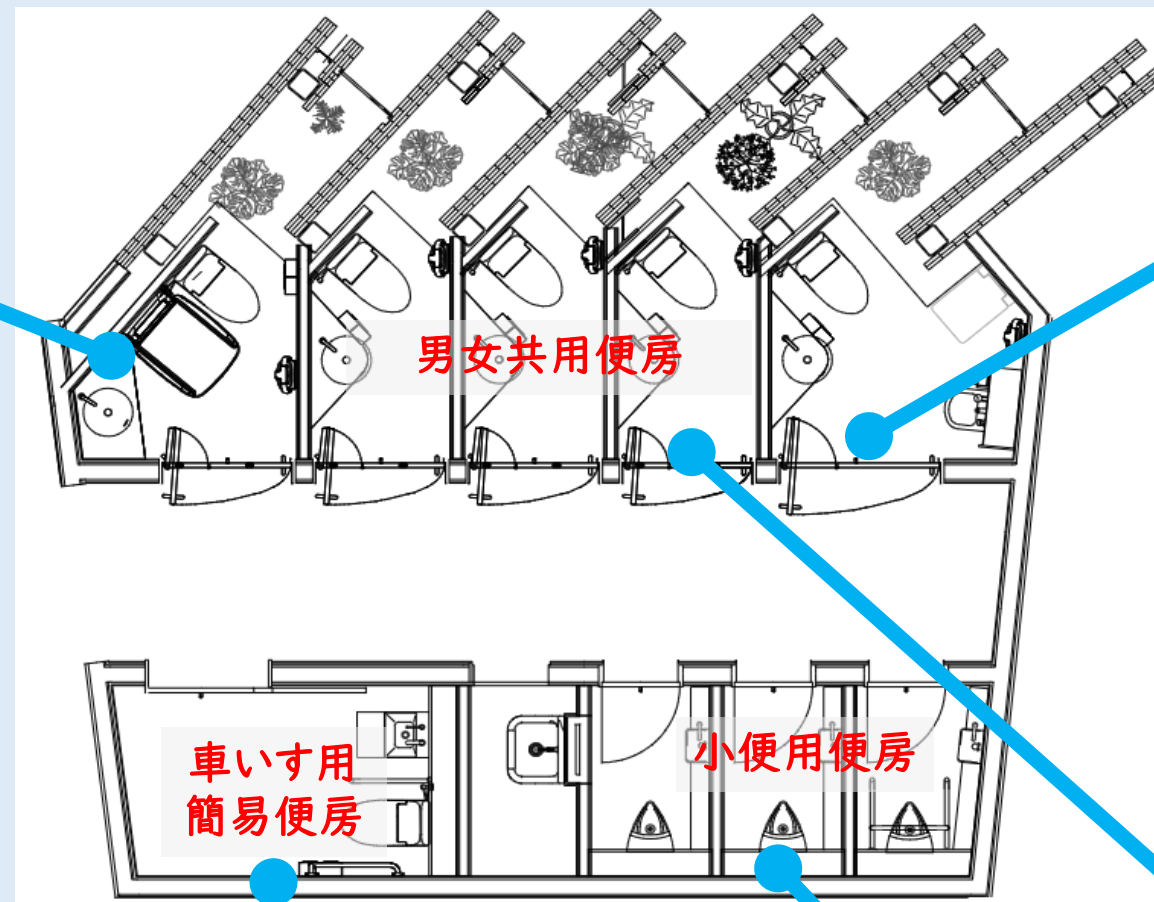
車いす用簡易便房
