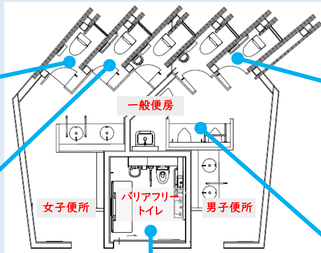
バリアフリートイレ
