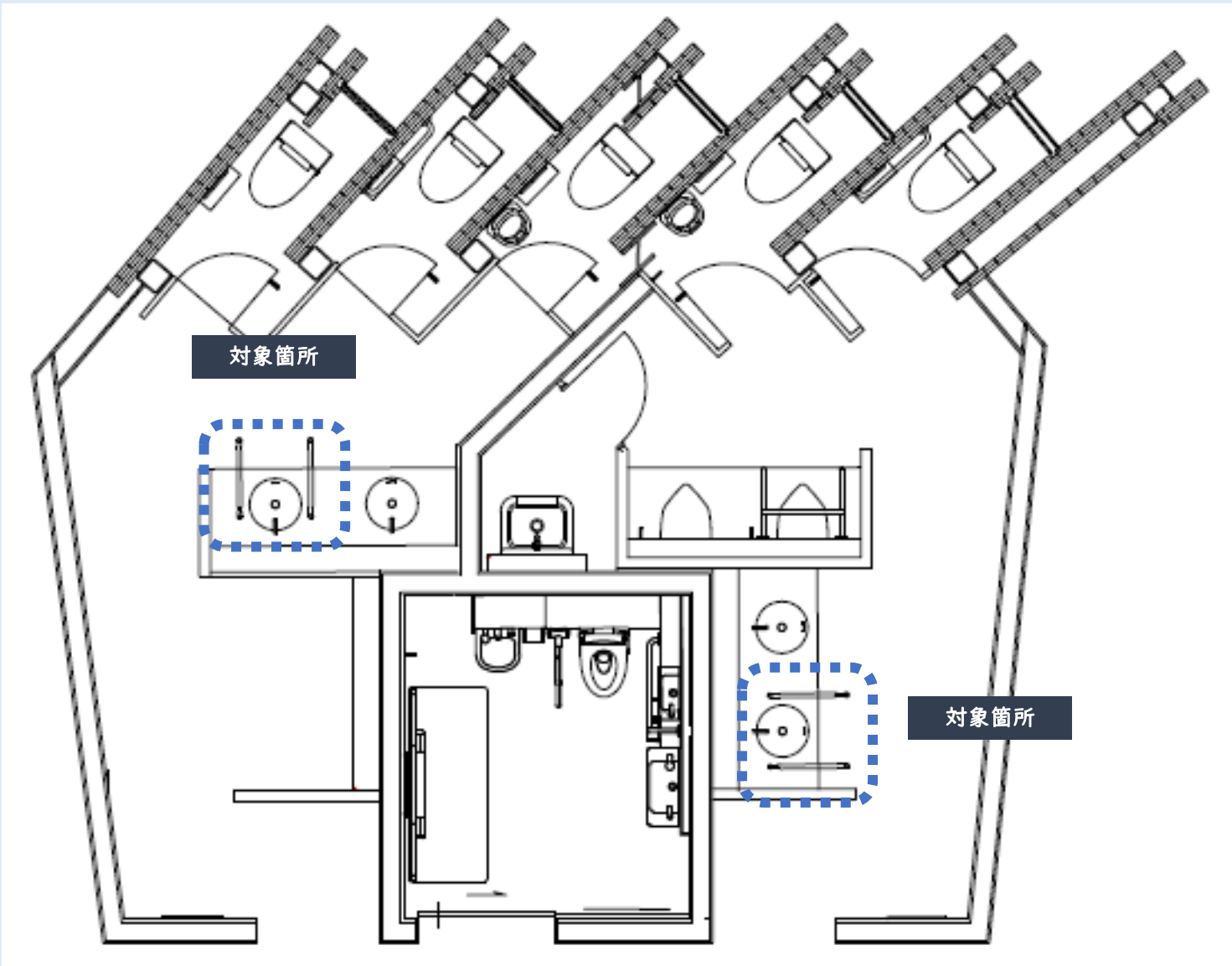
ゾーンA/C 従来型のトイレ
