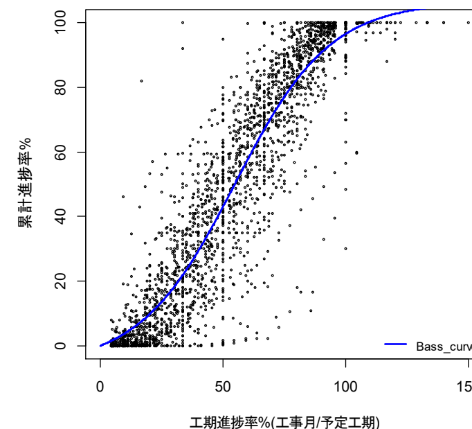
図2. Bassモデルによる進捗率曲線 1. 橋梁・高架構造物工事
