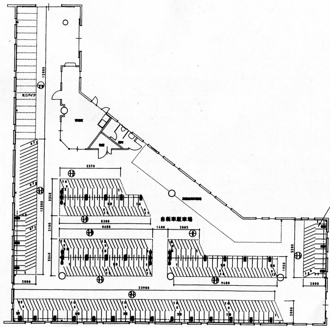
自転車駐車施設設備平面図 S-1:100
