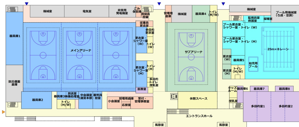
【1階平面図】
