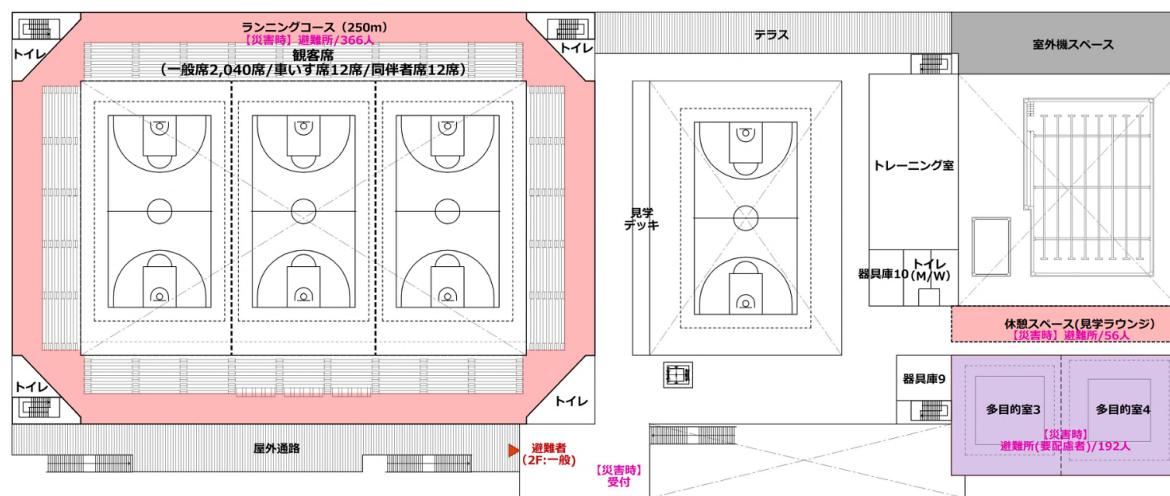
【2階平面図】
