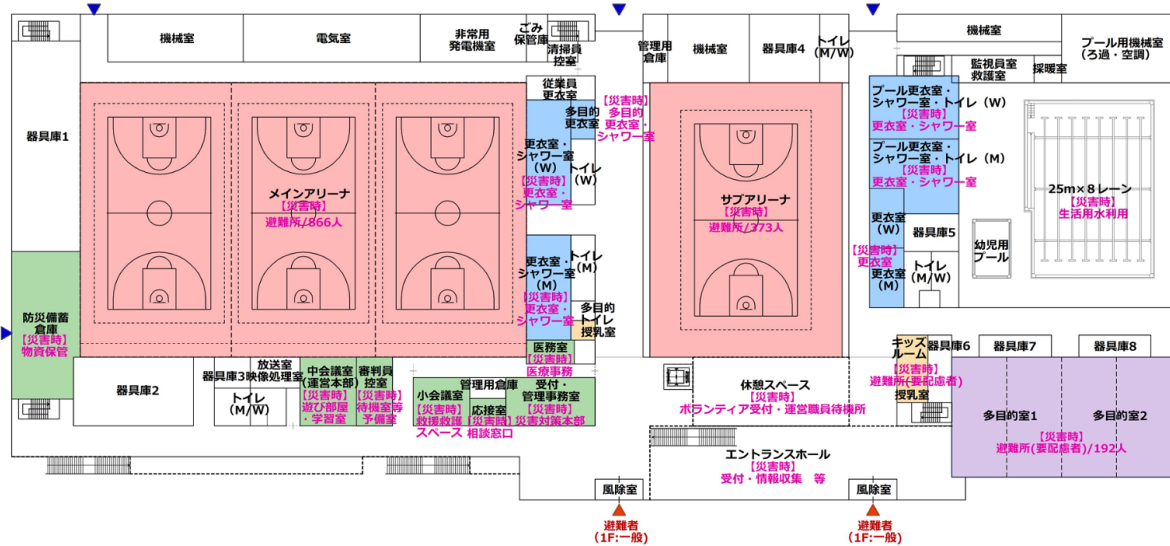
【1階平面図】
