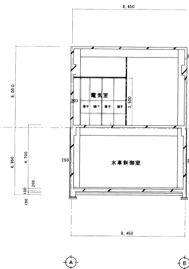
縦断面図 縮尺 1:100
