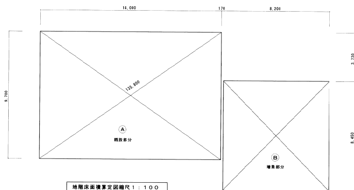
地階床面積算定図縮尺 1:100
