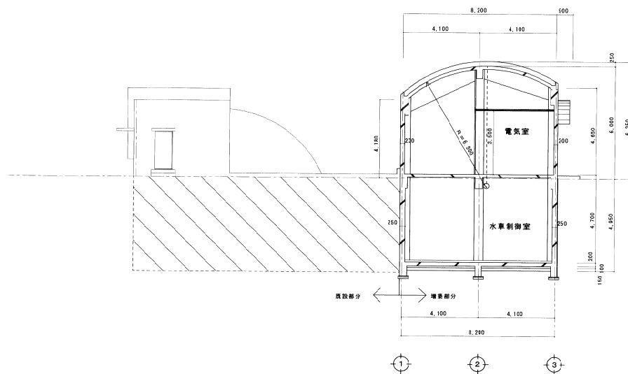
横断面図 縮尺 1:100
