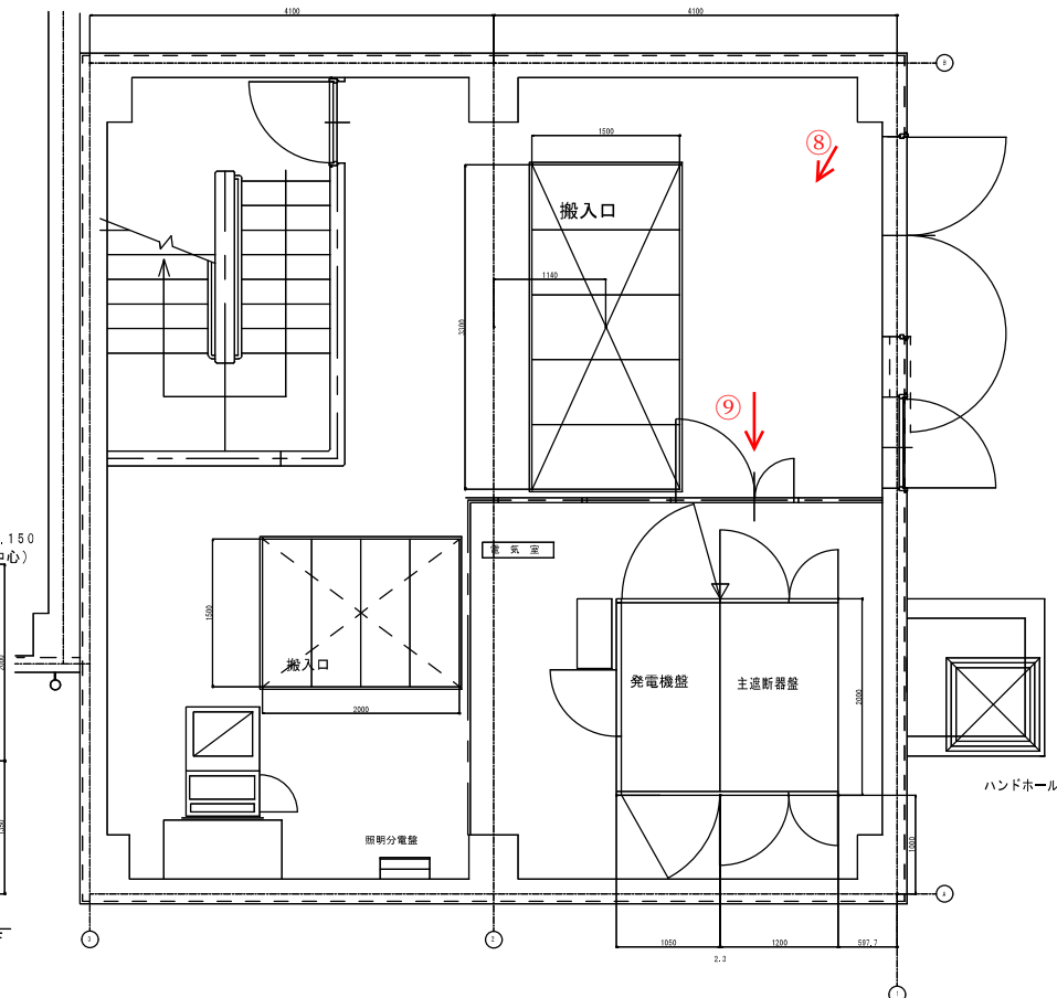
1FL 電気室配置
