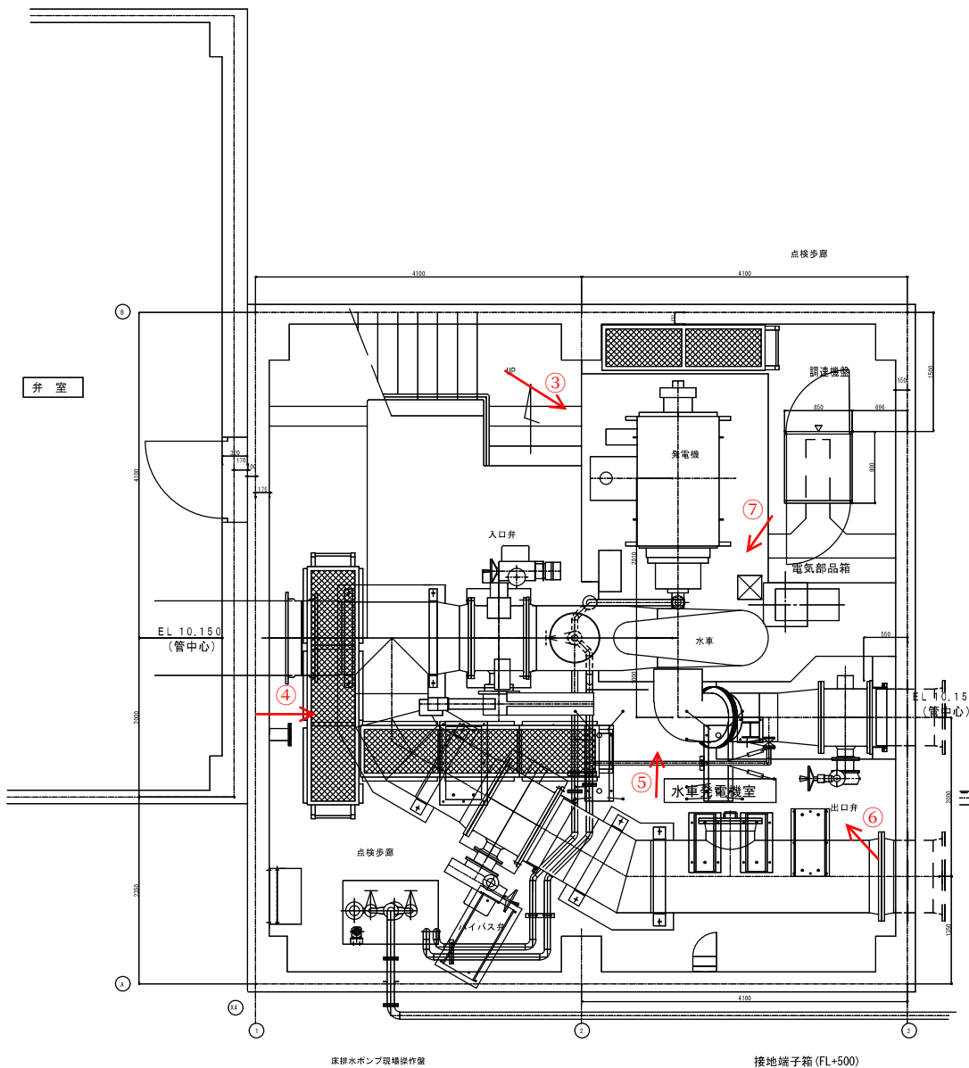
B1F 水車発電機室配置
