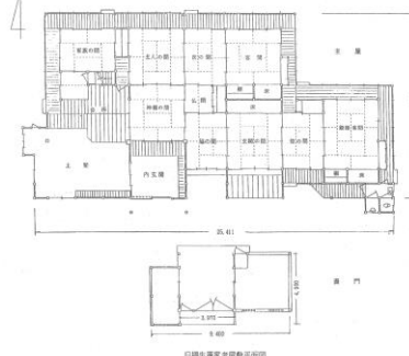
施設平面図
