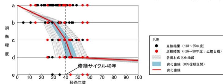
橋梁の点検結果を基にしたRC床版の劣化予測 (川崎市)
