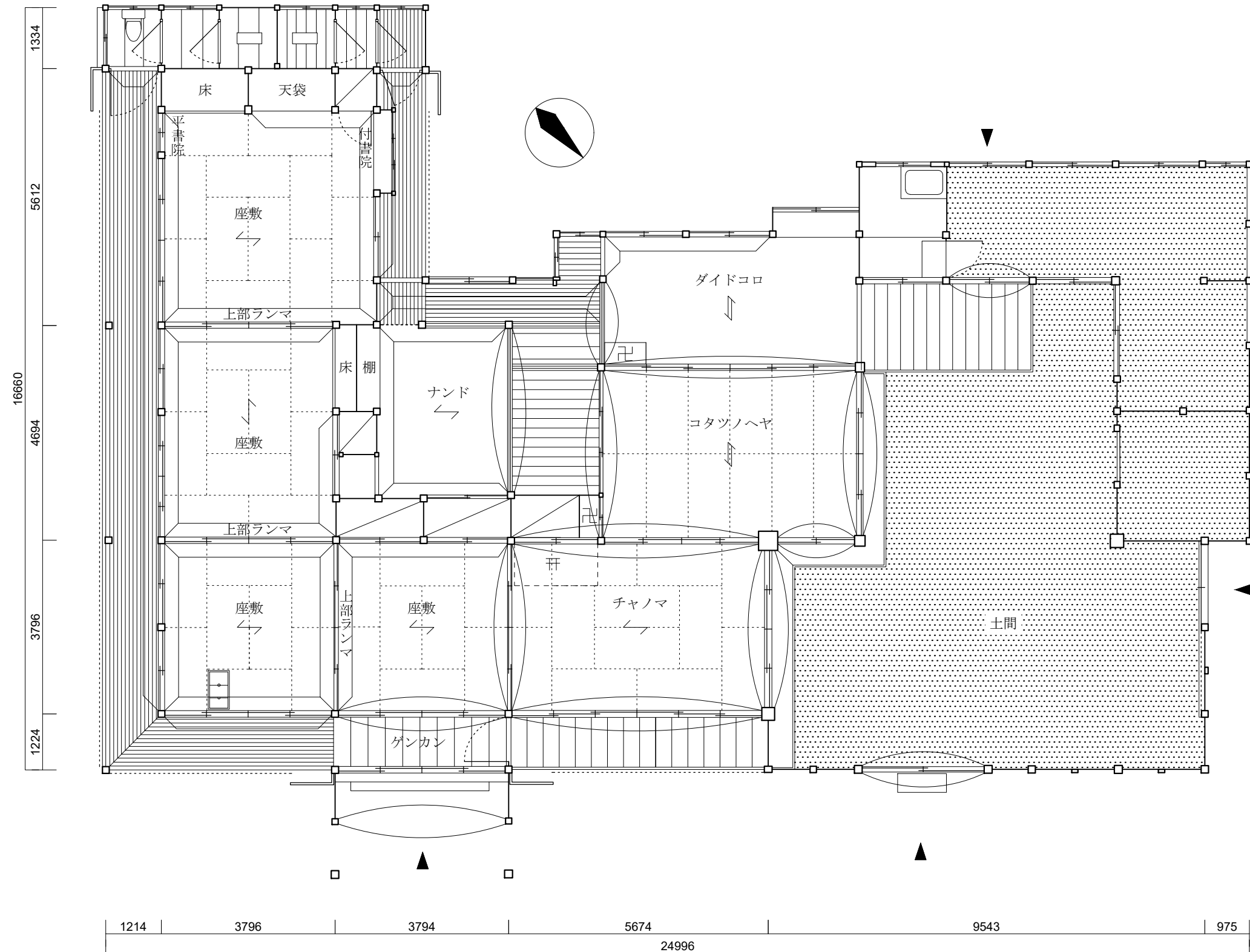
1 / 1 0 0 ・ 富田家住宅主屋平面図
