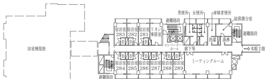
宿泊棟（A）2階平面図（510㎡）
