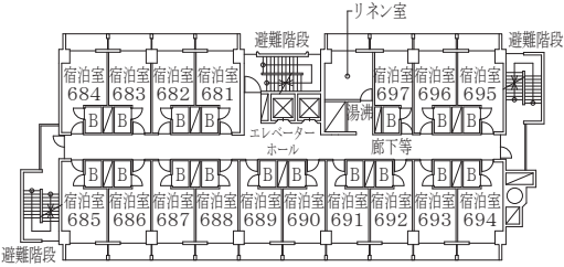
宿泊棟（Ａ）6階平面図（ 5 0 1 ㎡）
