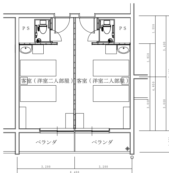
B・C棟宿泊室 洋室ツイン・トイレ付1／50
