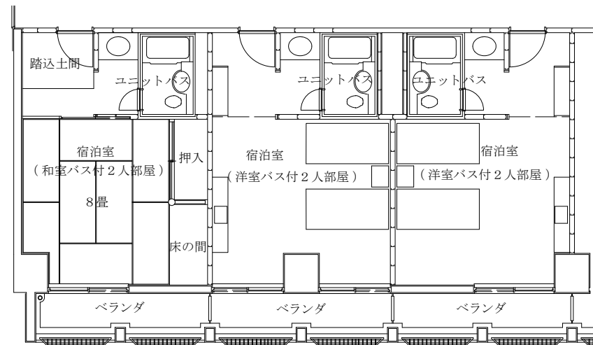
A棟宿泊室・和室ツイン・バストイレ付 1/50
