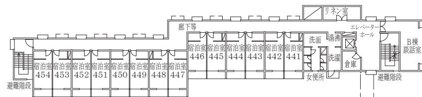
宿泊棟（B）4階平面図（599㎡）
