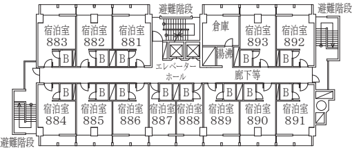
宿泊棟（Ａ）8階平面図（ 5 0 1 ㎡）
