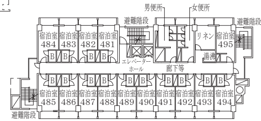
宿泊棟（A）4階平面図（501㎡）
