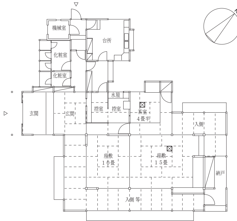
日本家屋 平面図 (198㎡) (響書院)
