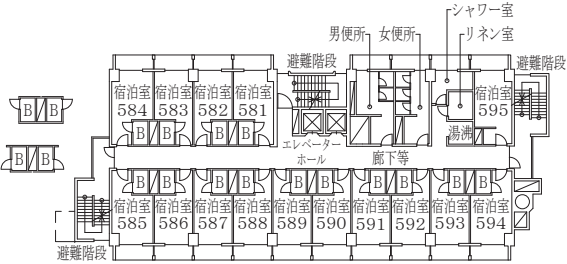
宿泊棟（Ａ）5階平面図（ 5 0 1 ㎡）
