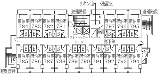
宿泊棟（Ａ）7階平面図（ 5 0 1 ㎡）
