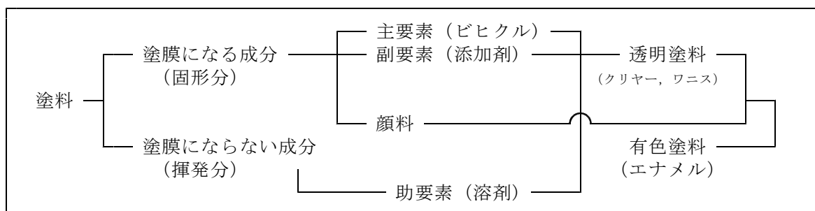
図2.2-1 塗料の構成
