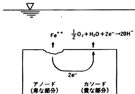
図2.1-1 電解質溶液中における鋼の腐食例
