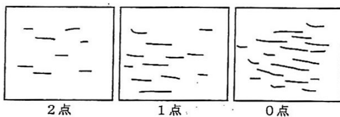
図5.3-2 われ評価図
