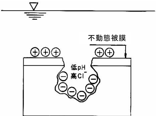
図2.1-2 孔食
