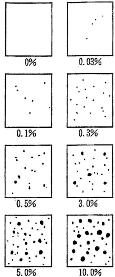
図5.3-1 さび、ふくれ評価図
