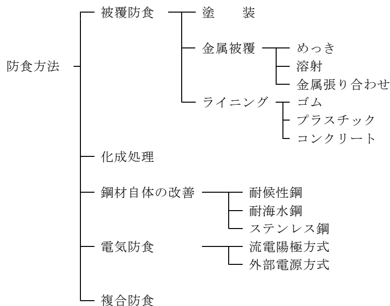
図3.1-1 防食方法の種類
