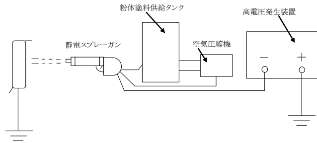
図4.2-1 静電吹付法
