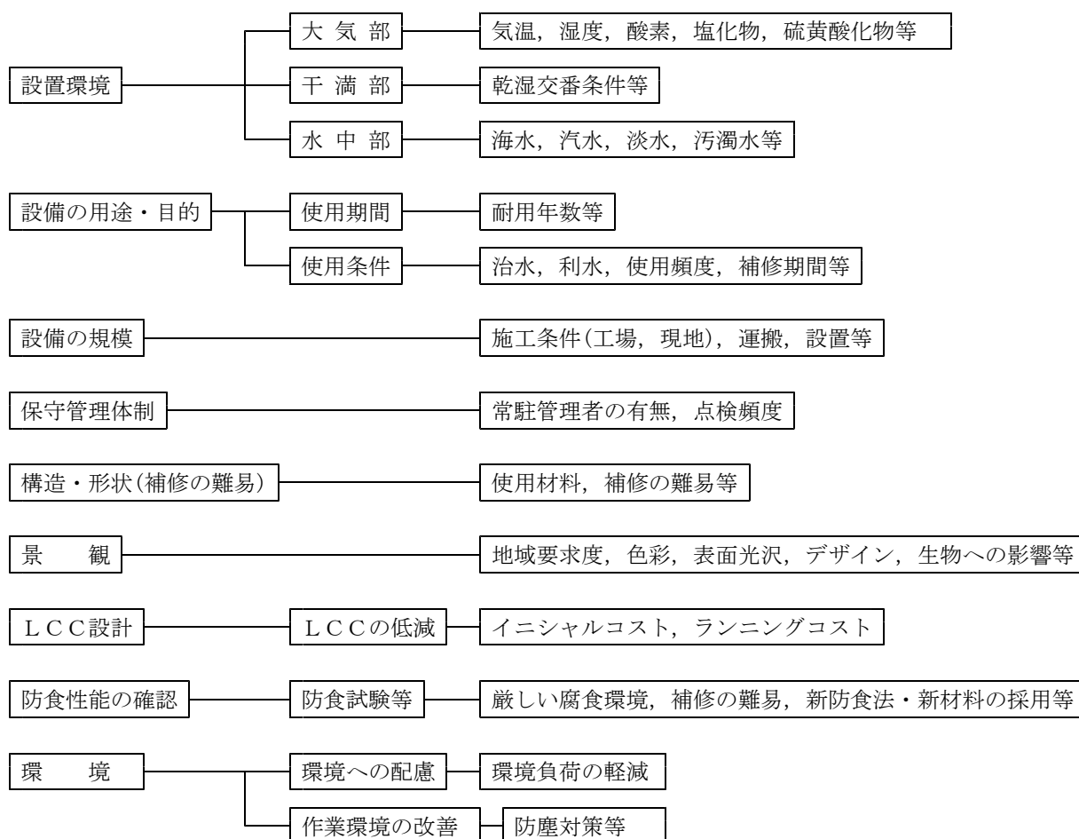
図3.1-2 防食設計における検討条件
